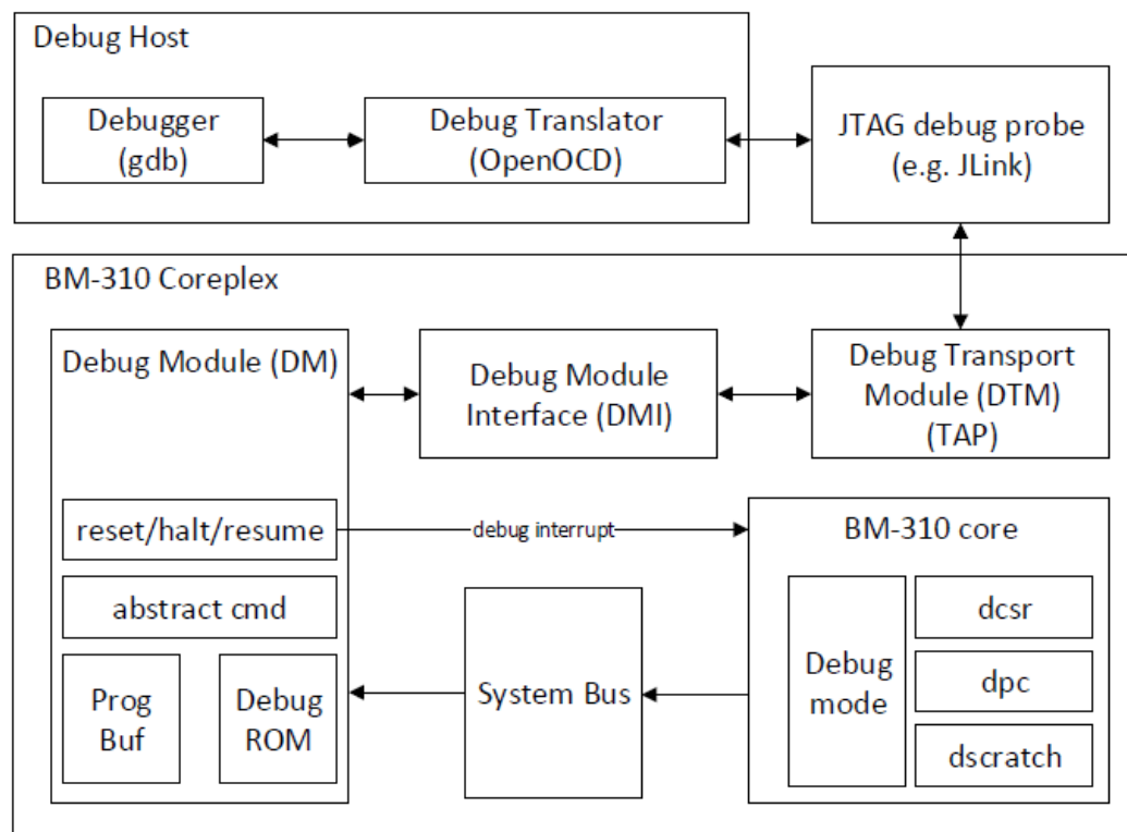
Рисунок 120 – Архитектура системы отладки
