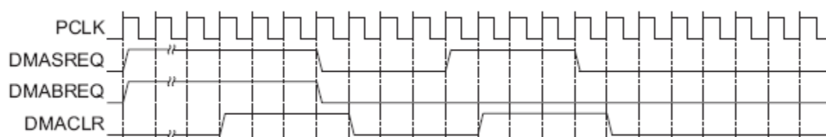
Рисунок 100 – Временные диаграммы обмена в режиме DMA
