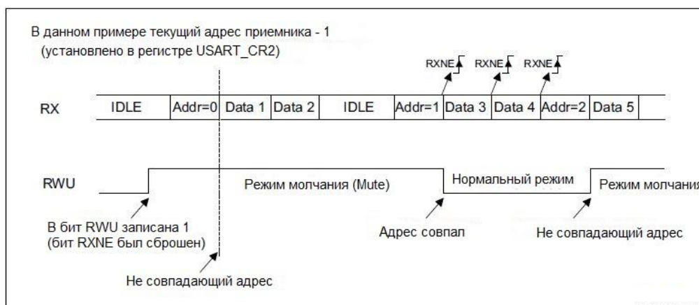
Рисунок 135 – Режим молчания (Mute) с обнаружением метки адреса
