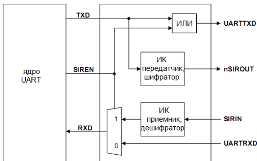
Рисунок 102 – Структурная схема кодека IrDA
