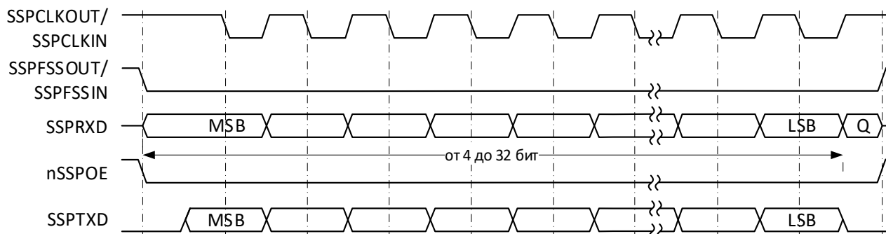
Рисунок 91 – Формат синхронного обмена протокола SPI, SPO=1, SPH=0 (одиночный обмен)
