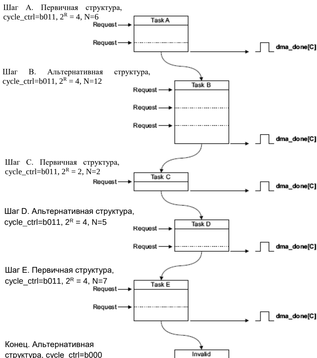
Рисунок 115 – Пример функционирования контроллера в режиме «пинг-понг»
