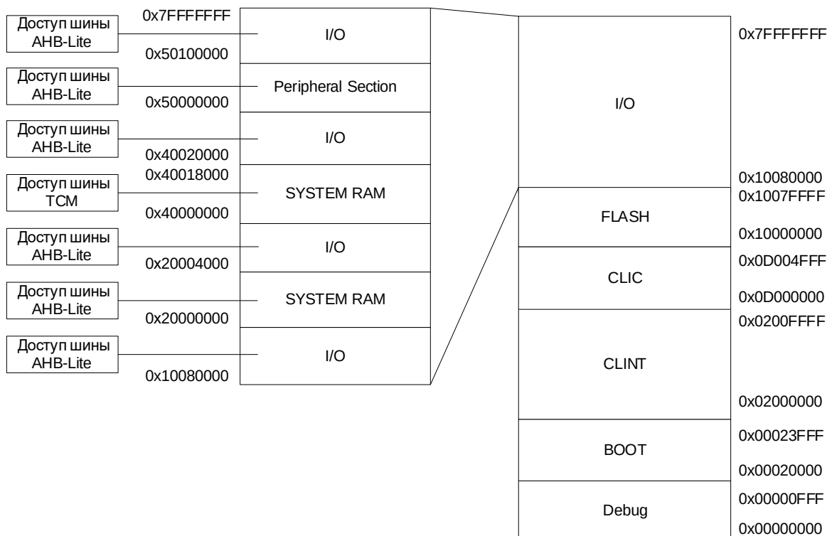
Рисунок 18 – Структура адресного пространства микросхемы
