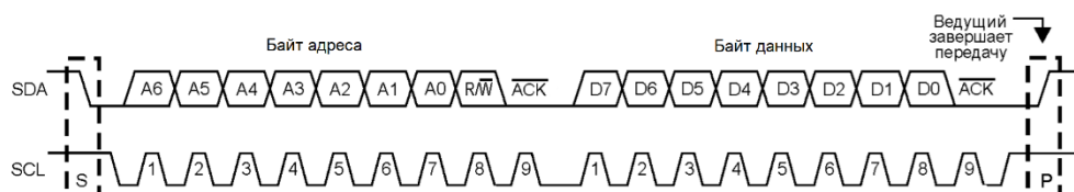
Рисунок 82 – Прием/передача по I2C в 7-битном режиме
