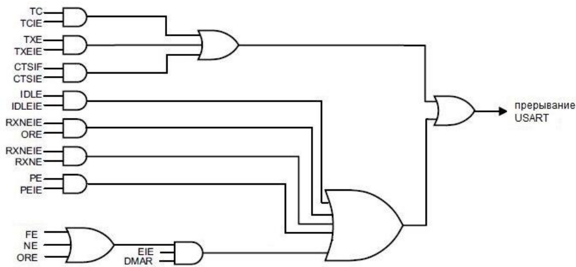
Рисунок 145 – Диаграмма отображений событий USART на прерывание
