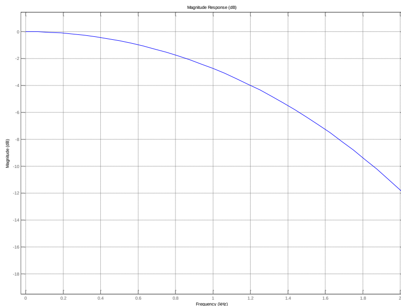
Рисунок 40 – Характеристика децимирующего фильтра в полосе 2 кГц при настройках по умолчанию
