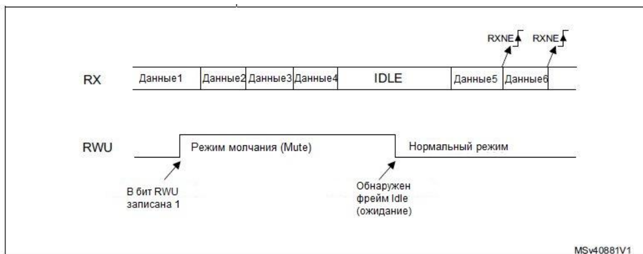
Рисунок 134 – Режим молчания (Mute) с обнаружением линии Idle
