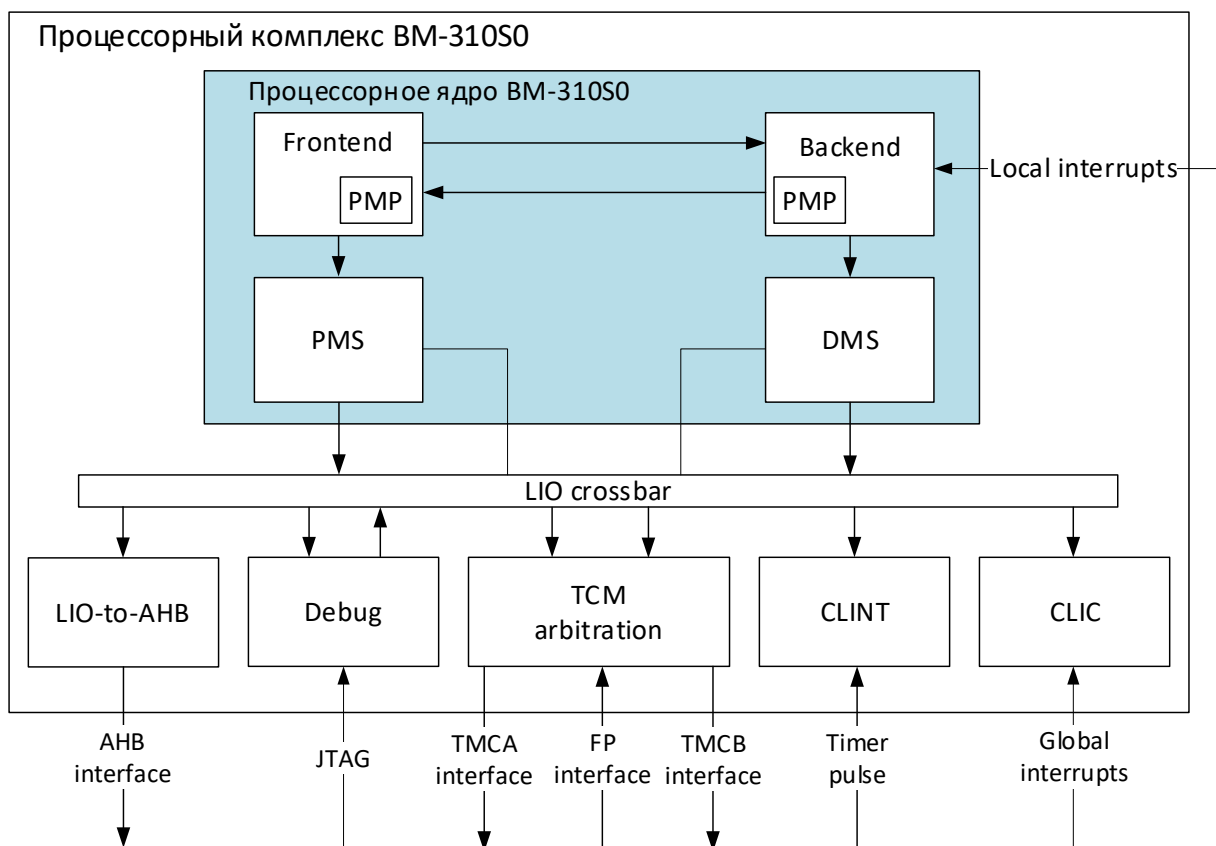
Рисунок 29 – Структурная схема процессора
