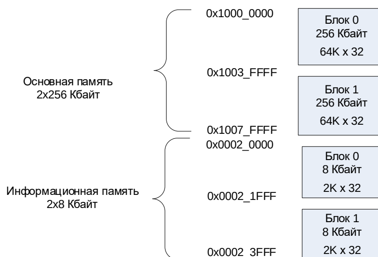
Рисунок 19 – Структура памяти
