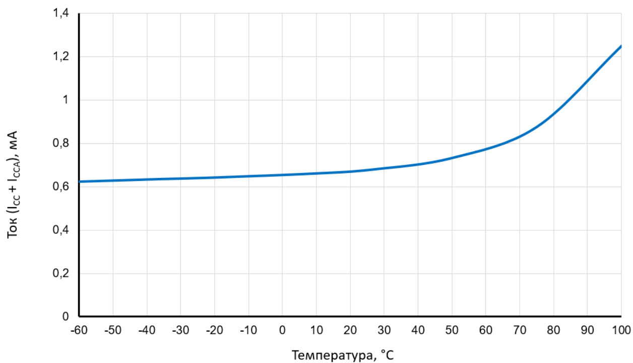
Рисунок 156 – Зависимость суммарного статического тока ( nRESET = 0 ) I_{CC} и I_{CCA} микросхем MDR1206FI (CHIP_ID = 217) от температуры при U_{CC} = U_{CCA} = 3,3 В
