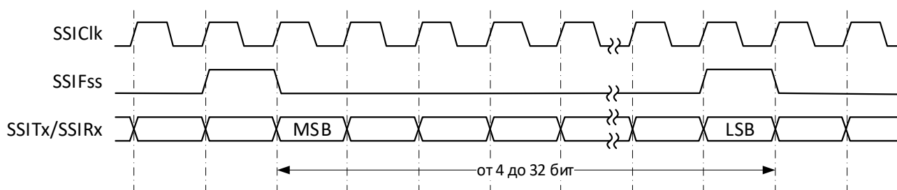
Рисунок 87 – Формат синхронного обмена протокола SSI (непрерывный обмен)
