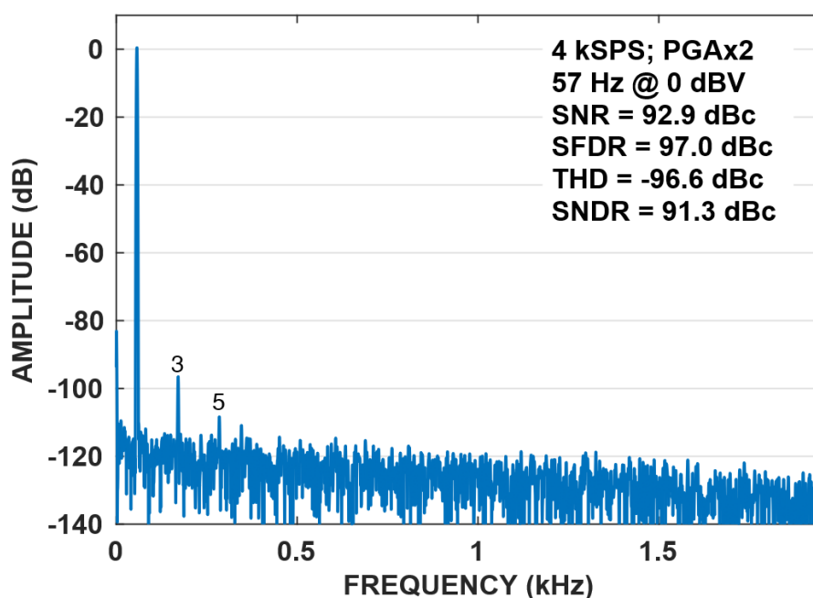
Рисунок 147 – Типовой спектр в НУ для \Delta\Sigma АПЦ микросхем MDR1206AFI (CHIP_ID = 215) в канале F2IDAT для дифференциального входного сигнала +/- 1 В (0.707 RMS). Усиление = 6 дБ (F2IGAIN = 00)
