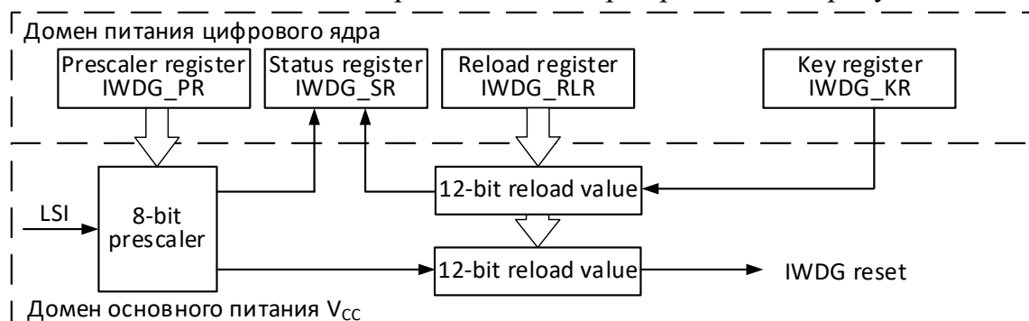
Рисунок 123 – Блок-схема независимого сторожевого таймера
