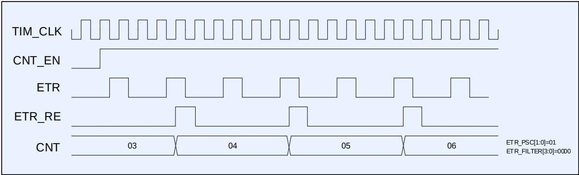
Рисунок 66 – Диаграмма тактирования со входа ETR, EVNT_SEL[3:0] = 1000
