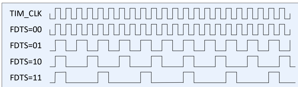
Рисунок 57 – Диаграмма тактовой частоты F_{DTS} в зависимости от значения FDTs[1:0] в регистре CNTRL
