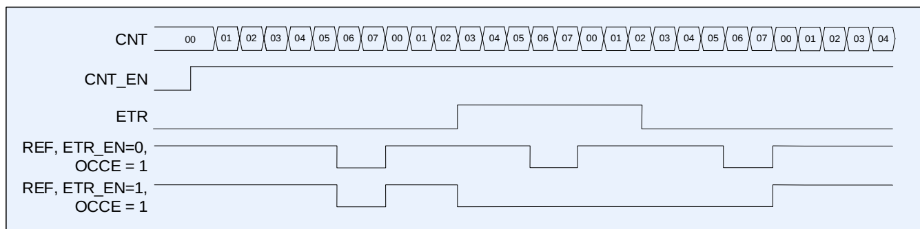
Рисунок 72 – Диаграмма сброса сигнала REF по выводу ETR
