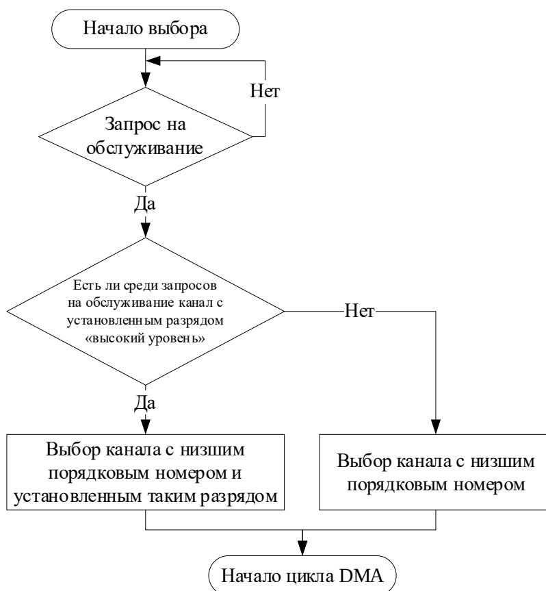
Рисунок 114 – Алгоритм выбора следующего канала для обслуживания
