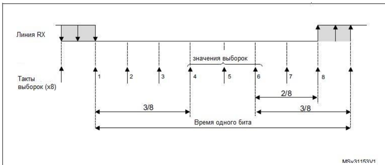
Рисунок 133 – Выборка данных при передискретизации на 8
