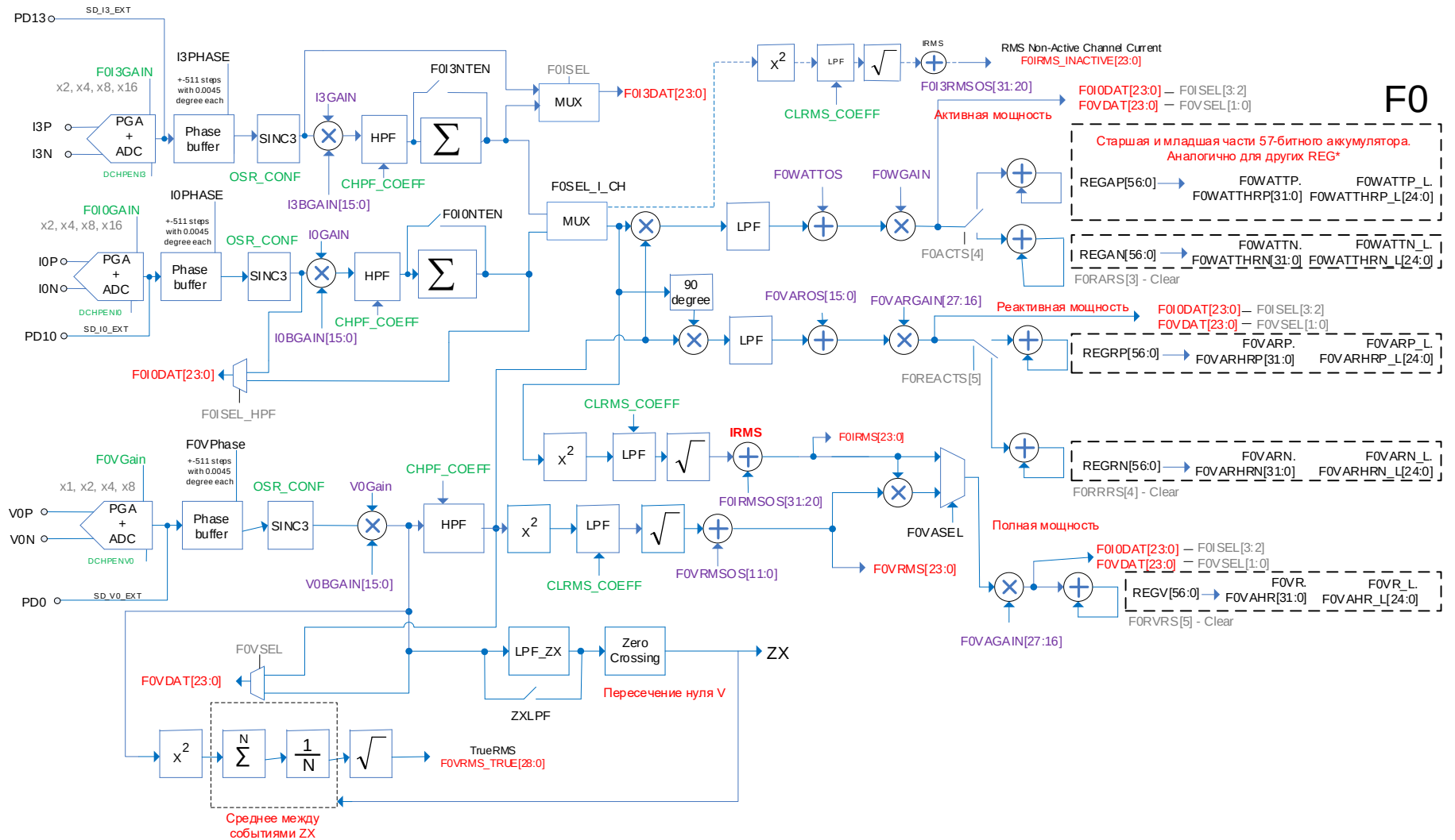
Рисунок 33 – Структурная схема F0
