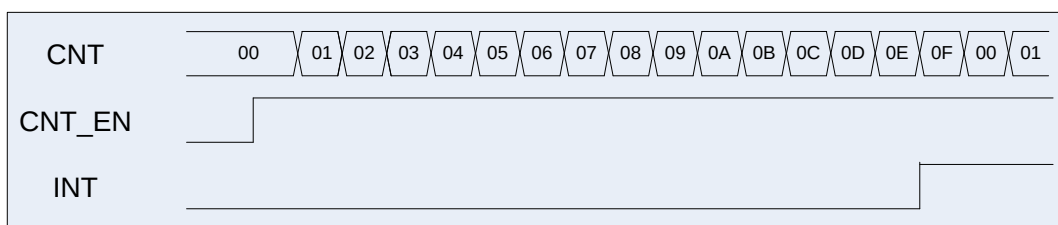
Рисунок 77 – Режим обычного счетчика
