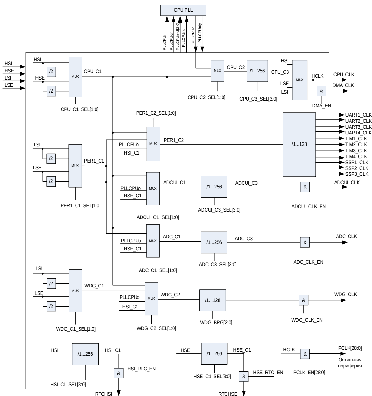
Рисунок 46 – Структурная блок-схема формирования тактовой частоты
