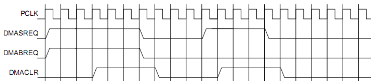
Рисунок 107 – Временные диаграммы одноэлементного и блочного запросов DMA
