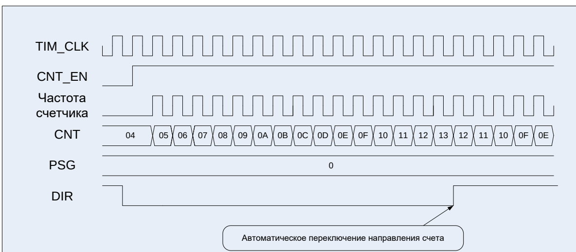
Рисунок 54 – Диаграммы работы таймера, счет двунаправленный, сначала прямой
