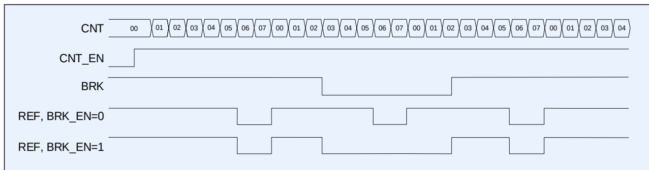
Рисунок 73 – Диаграмма сброса сигнала REF по выводу BRK
