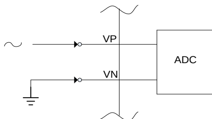
Рисунок 38 – Недифференциальное включение
