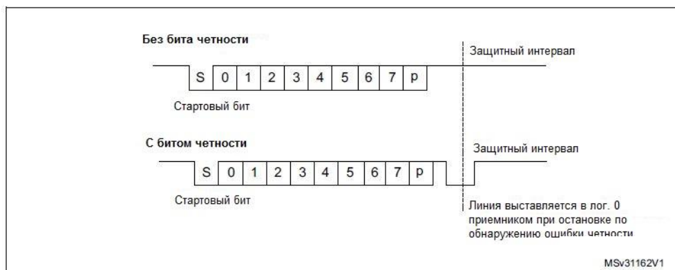
Рисунок 140 – Асинхронный протокол ISO 7816-3
