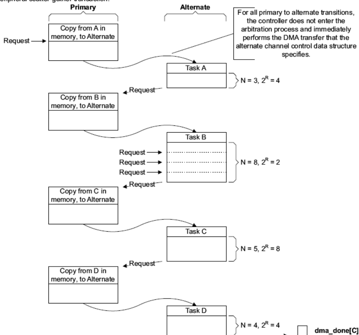
Рисунок 117 – Пример работы DMA в режиме с «Исполнением с изменением конфигурации»
