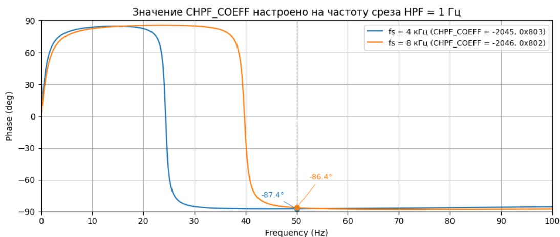
Рисунок 32 – ФЧХ интегратора для частот дискретизации 4 и 8 кГц (при 16 кГц работа интегратора не гарантируется)
