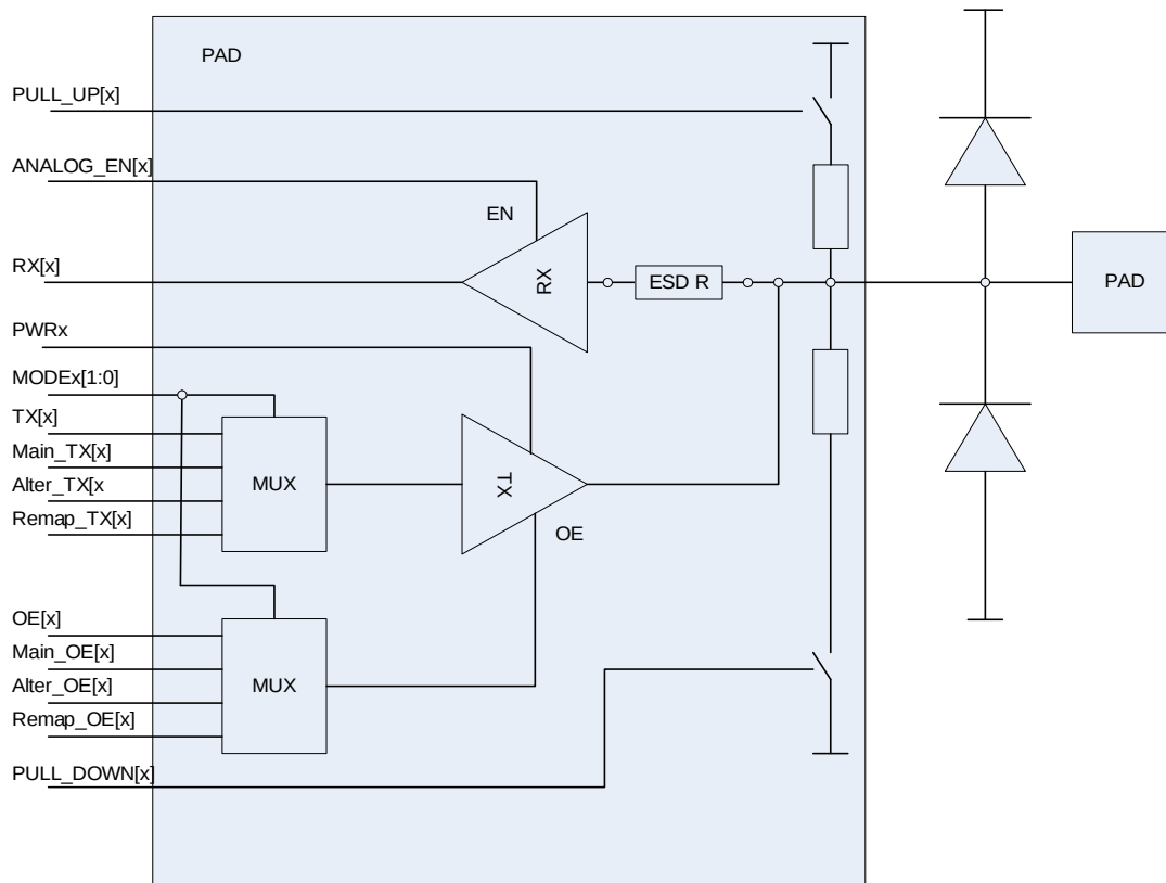
Рисунок 50 – Блок схема разряда порта ввода-вывода
