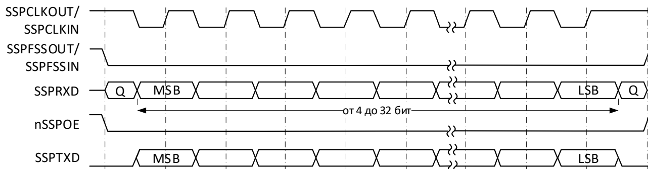
Рисунок 93 – Формат синхронного обмена протокола SPI, SPO=1, SPH=1
