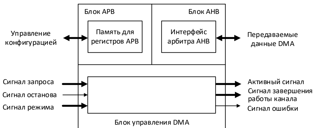
Рисунок 108 – Структурная схема контроллера
