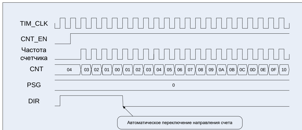
Рисунок 55 – Диаграммы работы таймера, счет двунаправленный, сначала обратный
