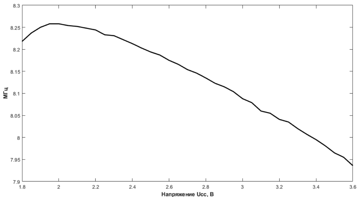
Рисунок 153 – Зависимость частоты RC генератора HSI микросхем MDR1206FI, MDR1215LGI (CHIP_ID = 217) от напряжения питания U_{CC} в НУ
