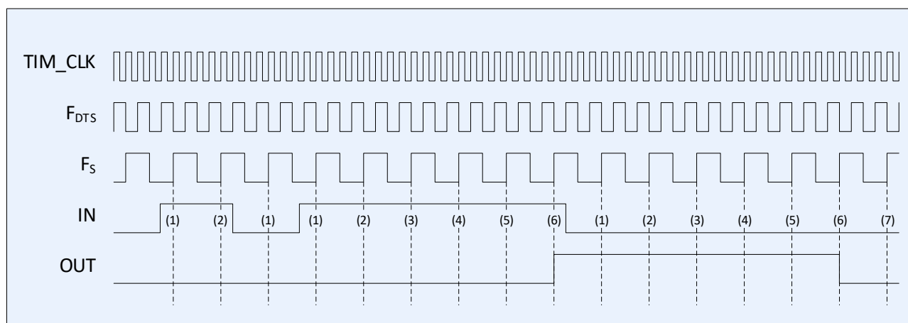
Рисунок 76 – Диаграмма работы фильтра, F_S = F_{DTS}/2 , N = 6
