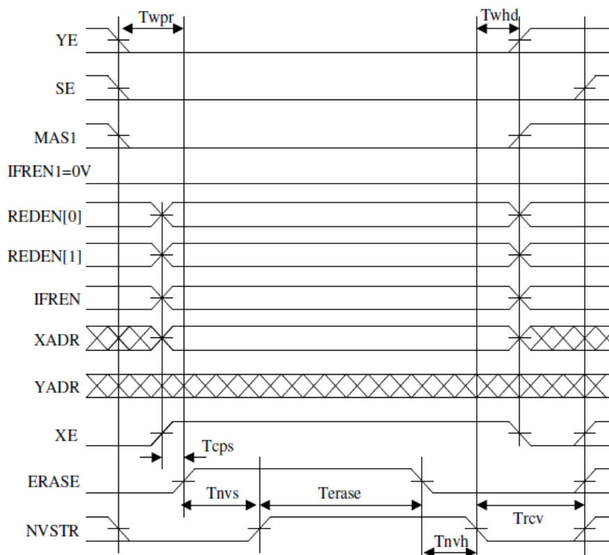
Рисунок 21 – Временная диаграмма стирания страницы памяти
