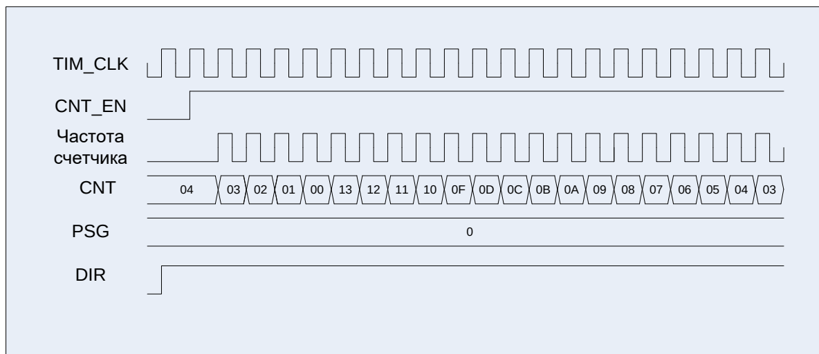
Рисунок 53 – Диаграммы работы таймера, счет обратный от 0x13 до 0, стартовое значение 0x04
