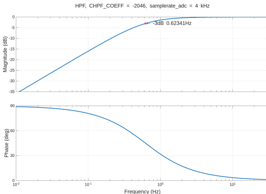
Рисунок 30 – ЛАЧХ и ФЧХ фильтра HPF при настройках по умолчанию на 4 кГц
