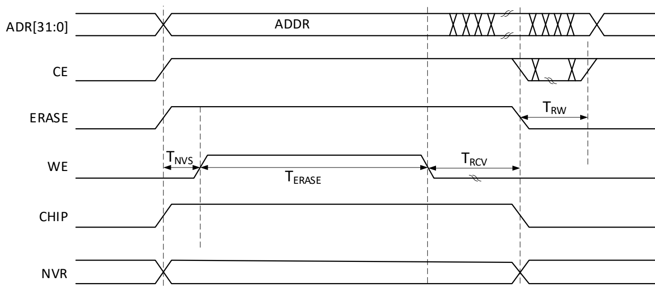
Рисунок 25 – Временная диаграмма стирания памяти
