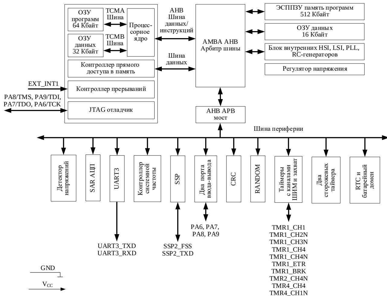
Рисунок 3 – Структурная блок-схема микросхем MDR1219LGI
