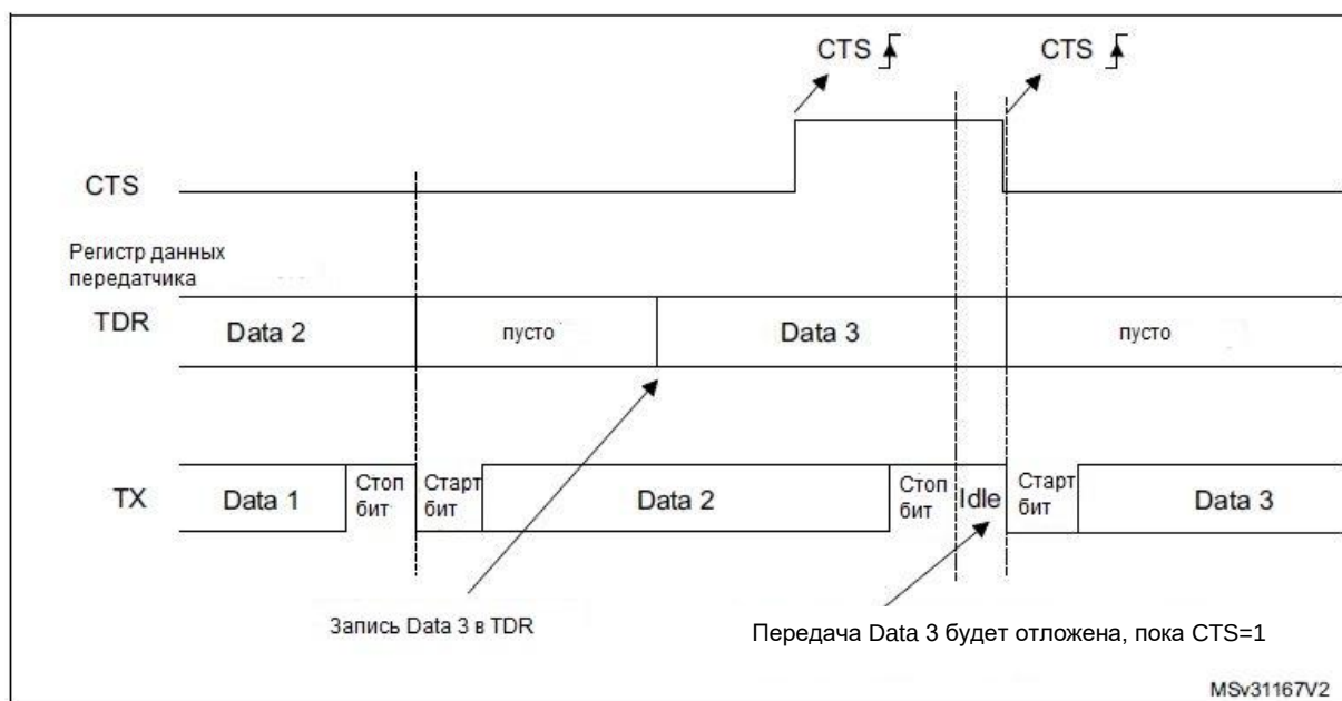
Рисунок 144 – Управление потоком CTS
