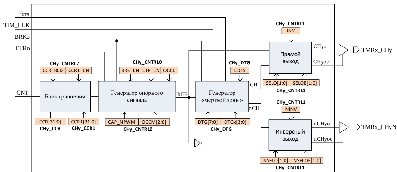
Рисунок 69 – Структурная схема блока формирования ШИМ
