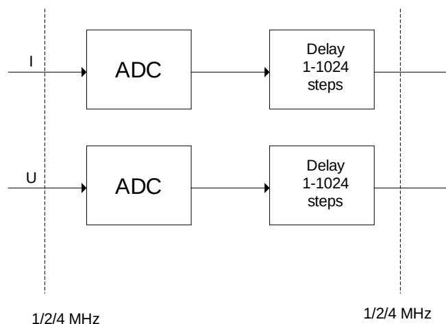
Рисунок 39 – Контролируемый фазовый сдвиг в каналах тока и напряжения
