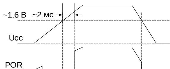
Рисунок 14 – Диаграмма формирования сигнала сброса микросхемы
