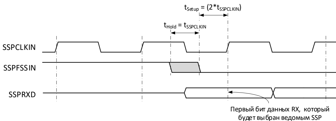
Рисунок 96 – Формат Microwire, требования к времени установки и удержания сигнала SSPFSSIN
