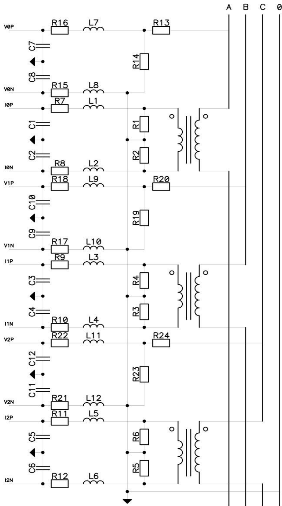
Рисунок 43 – Типовая схема включения для учета электроэнергии по трем фазам
