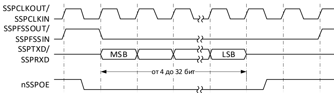
Рисунок 86 – Формат синхронного обмена протокола SSI (единичный обмен)
