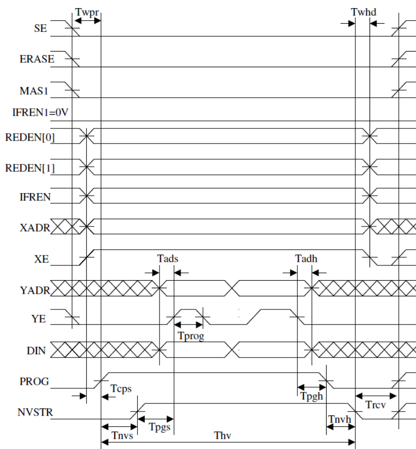
Рисунок 22 – Временная диаграмма записи памяти
