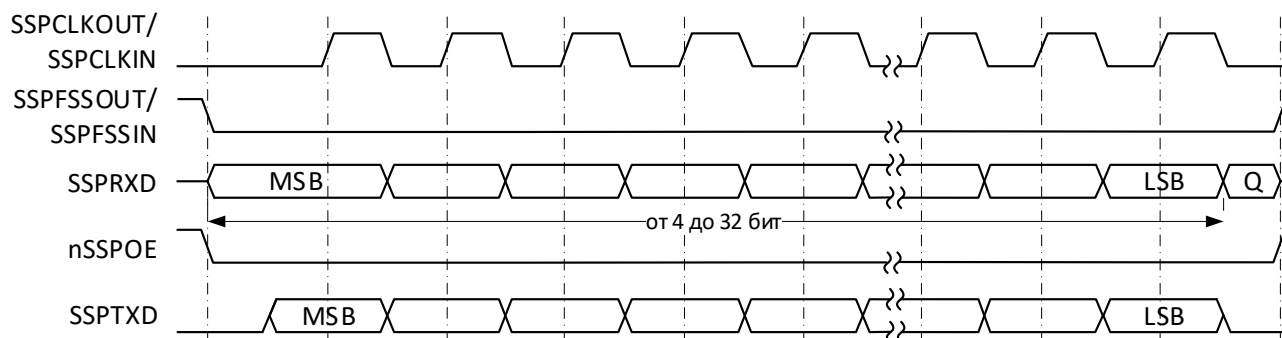
Рисунок 88 – Формат синхронного обмена протокола SPI, SPO=0, SPH=0 (одиночный обмен)
