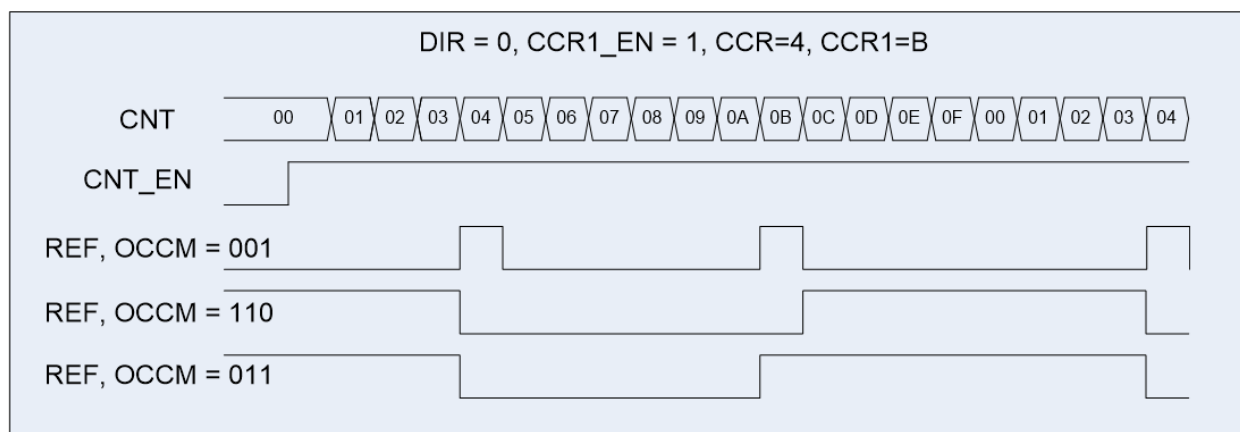
Рисунок 71 – Диаграмма работы в режиме ШИМ, CCR1_EN = 1
