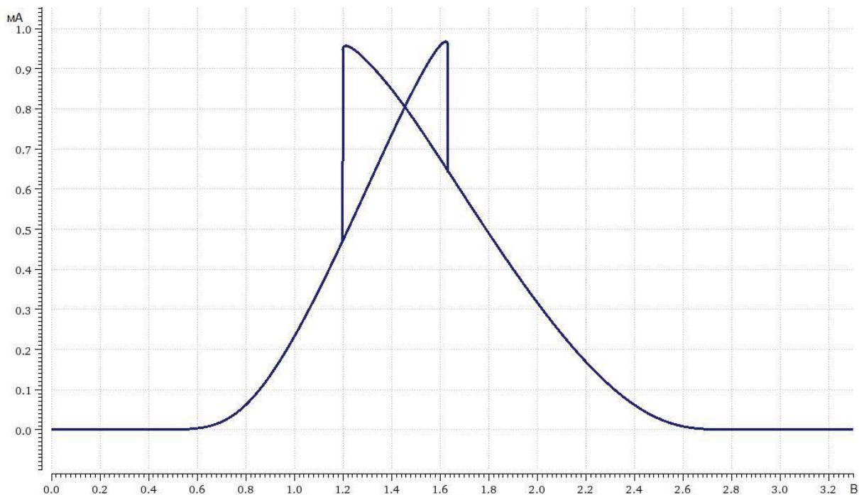
Рисунок 149 – Типовая зависимость дополнительного тока потребления по питанию U_{CC} от напряжения на цифровом входе порта ввода-вывода при U_{CC} = 3,3 В в НУ
