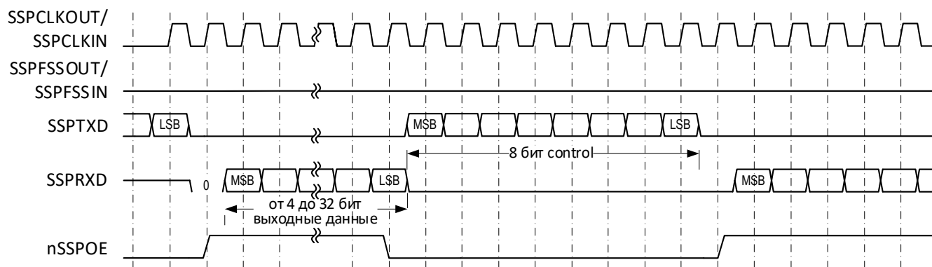
Рисунок 95 – Формат синхронного обмена протокола Microwire (непрерывный обмен)
