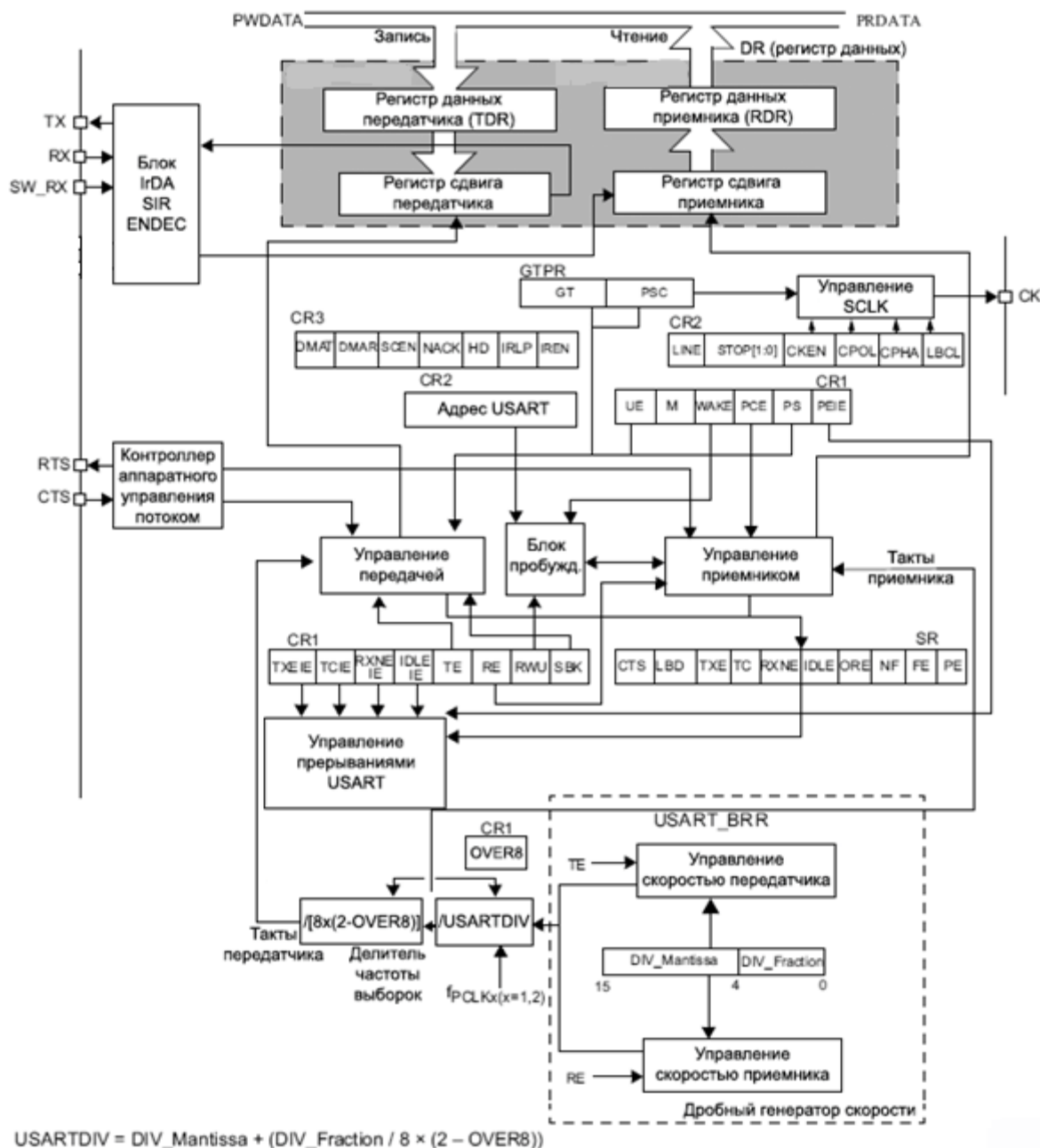
Рисунок 127 – Блок схема USART
