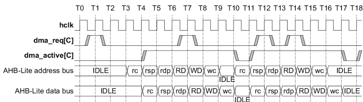
Рисунок 109 – Диаграмма работы при получении импульсного запроса от периферийного блока
