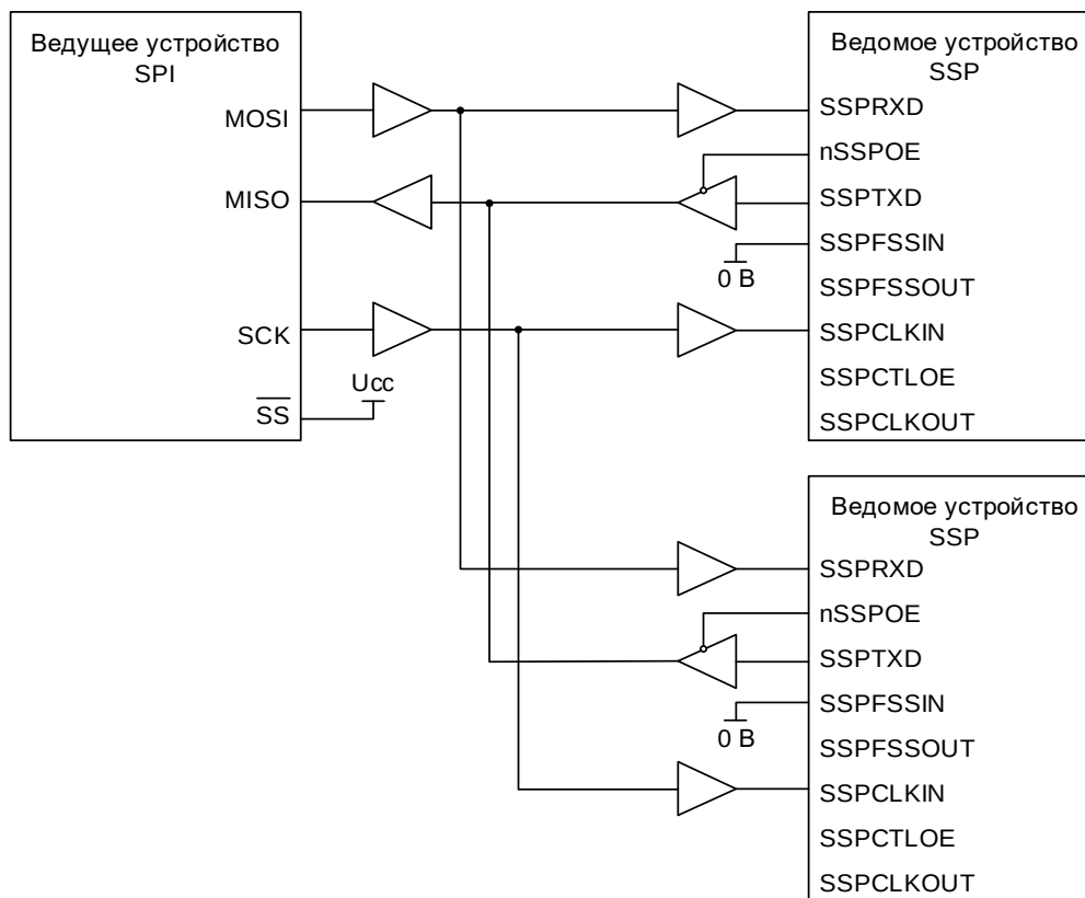
Рисунок 99 – Ведущее устройство, протокол SPI, подключено к двум ведомым модулям SSP
