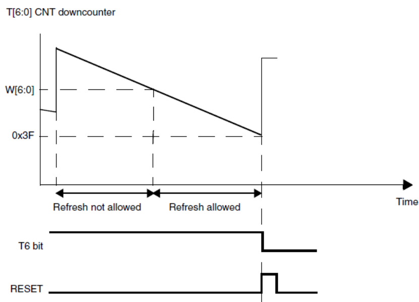
Рисунок 125 – Временная диаграмма оконного сторожевого таймера
