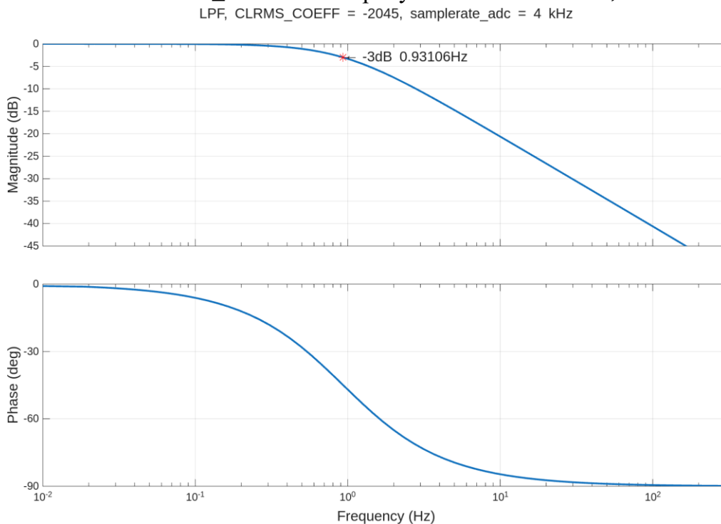
Рисунок 31 – ЛАЧХ и ФЧХ фильтра LPF при настройках по умолчанию на 4 кГц
