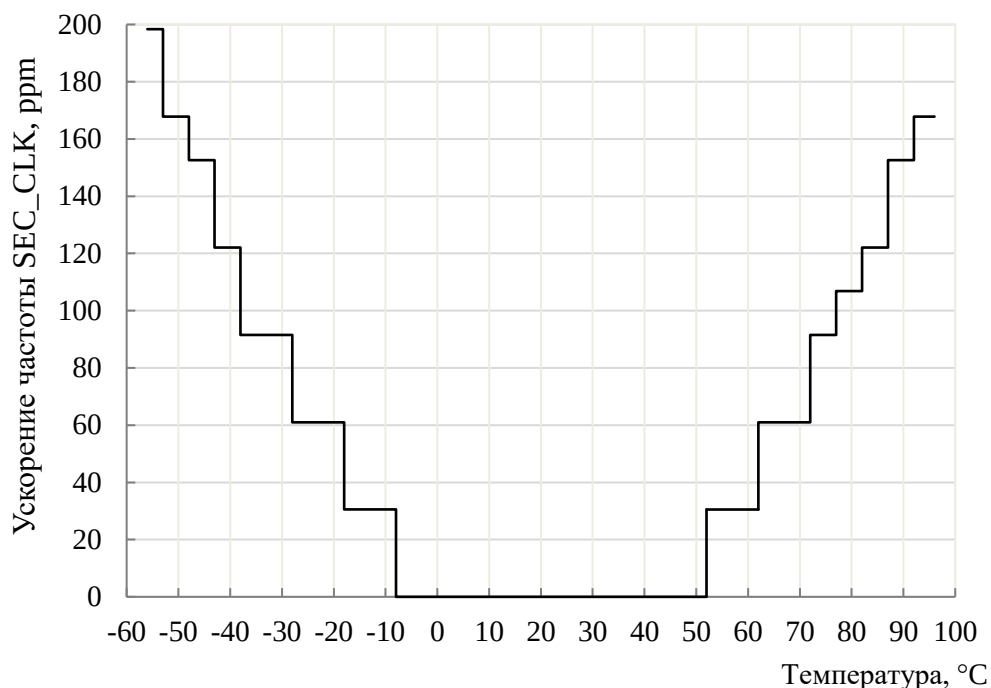
Рисунок 48 – Типовая зависимость поправки (ускорения) частоты SEC_CLK при BKP_RTC_PRL = 32767 от температуры
