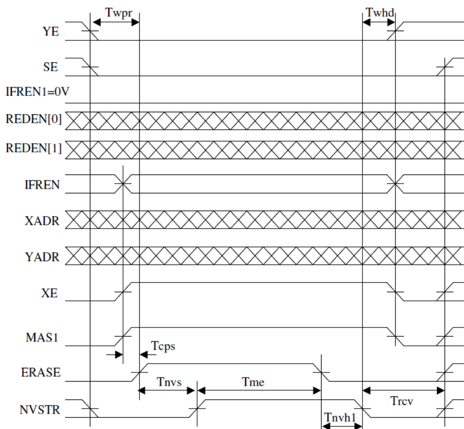
Рисунок 20 – Временная диаграмма стирания памяти
