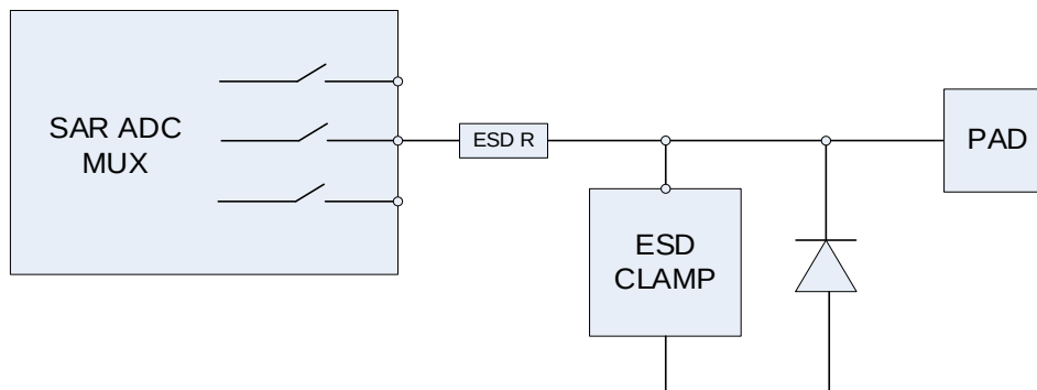
Рисунок 81 – Структурная схема выводов SAR_AINx
