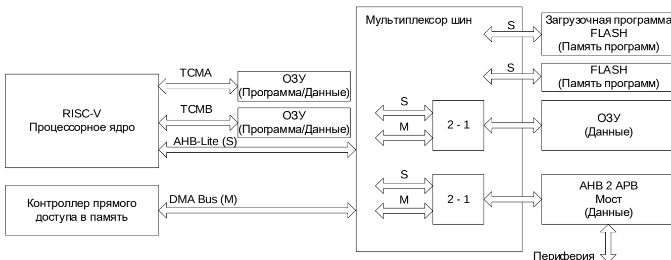
Рисунок 17 – Структурная схема организации памяти
