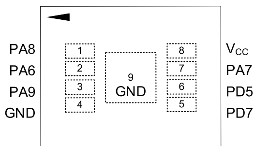
Рисунок 8 – Диаграмма расположения выводов микросхем MDR1215LGI
