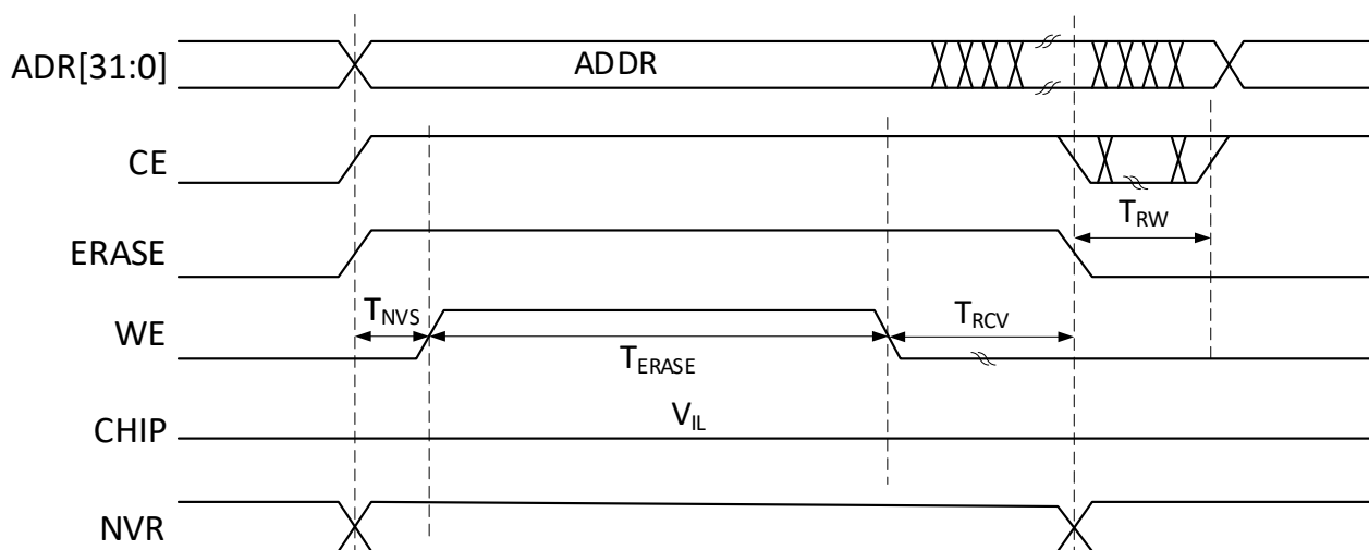
Рисунок 26 – Временная диаграмма стирания страницы памяти
