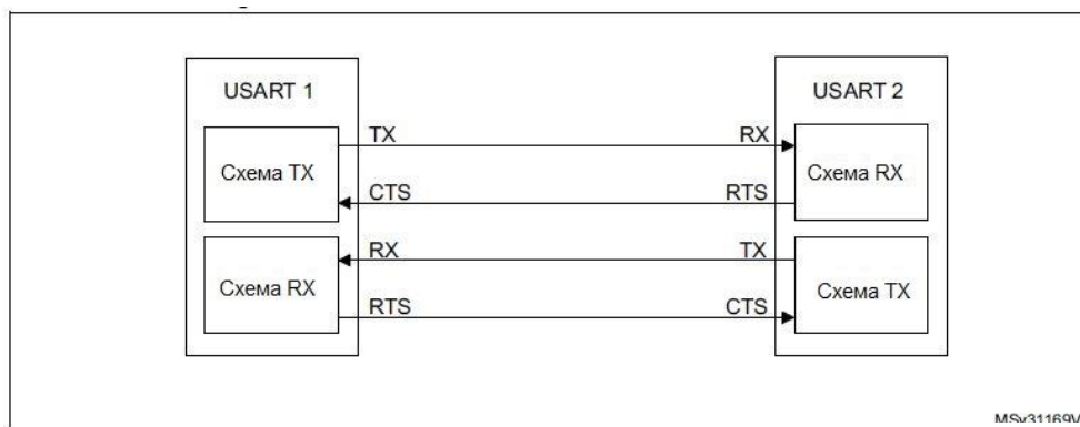
Рисунок 142 – Аппаратное управление потоком данных между двумя устройствами USART
