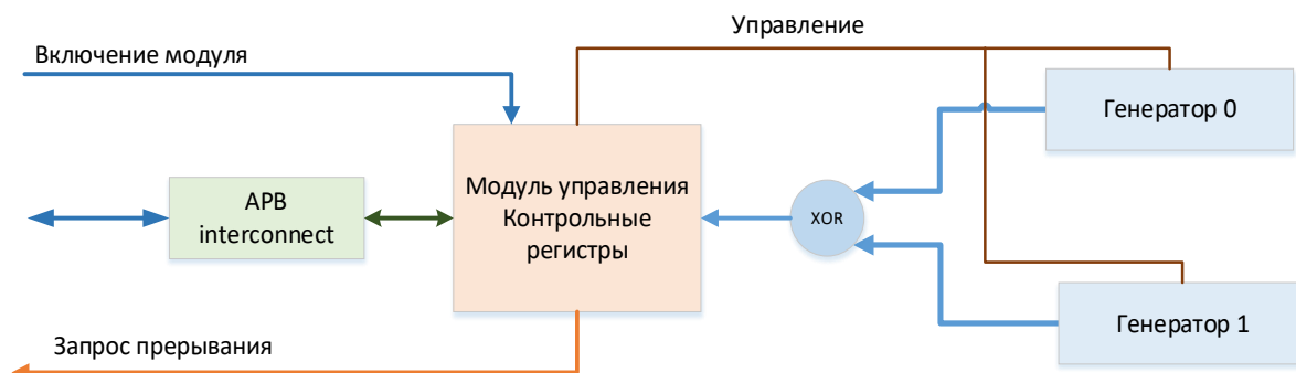
Рисунок 126 – Структурная схема блока генератора случайных чисел
