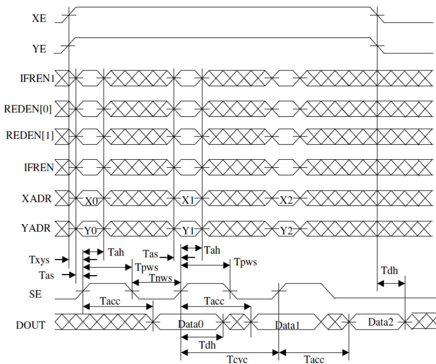
Рисунок 23 – Временная диаграмма чтения памяти
