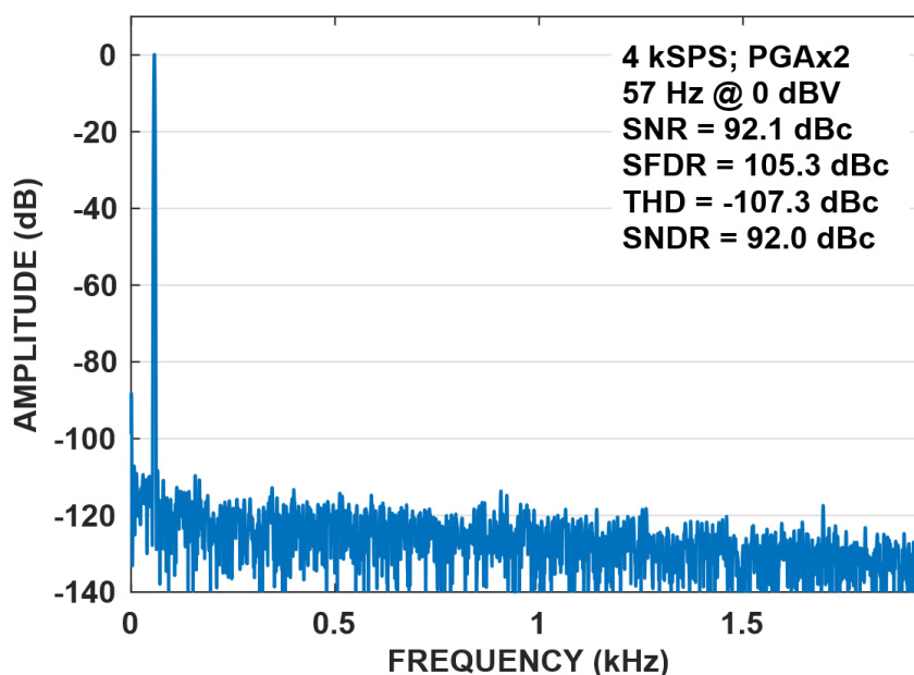
Рисунок 146 – Типовой спектр в НУ для \Delta\Sigma АЦП микросхем MDR1206FI (CHIP_ID = 217) в канале F2IDAT для дифференциального входного сигнала +/- 1 В (0.707 RMS). Усиление = 6 дБ (F2IGAIN = 00)
