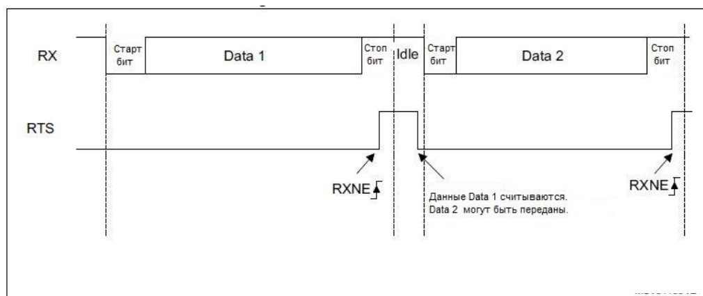
Рисунок 143 – Управление потоком RTS
