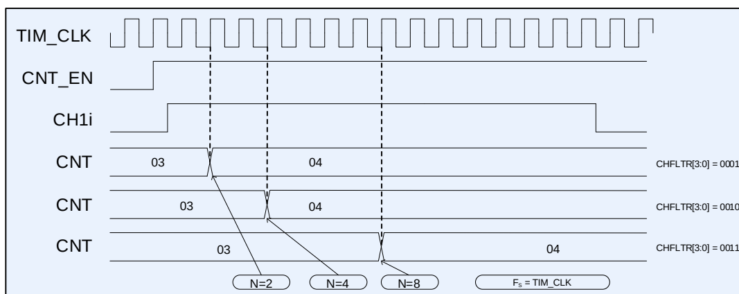
Рисунок 64 – Диаграмма внешнего тактирования с разными вариантами фильтра
