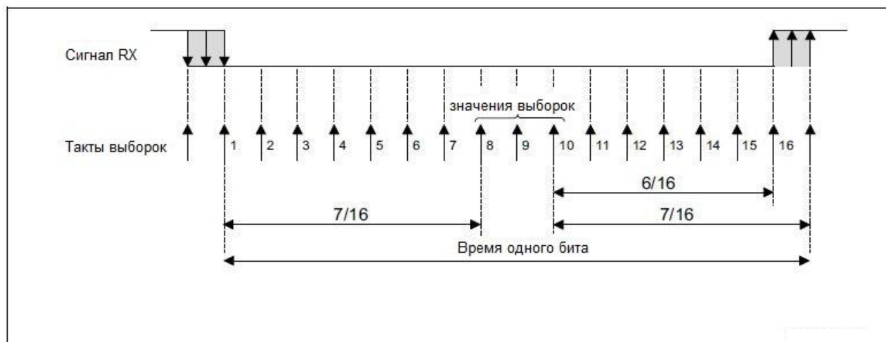
Рисунок 132 – Выборка данных при передискретизации на 16
