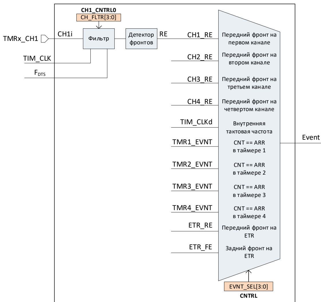
Рисунок 63 – Схема тактирования сигналом со входа первого канала
