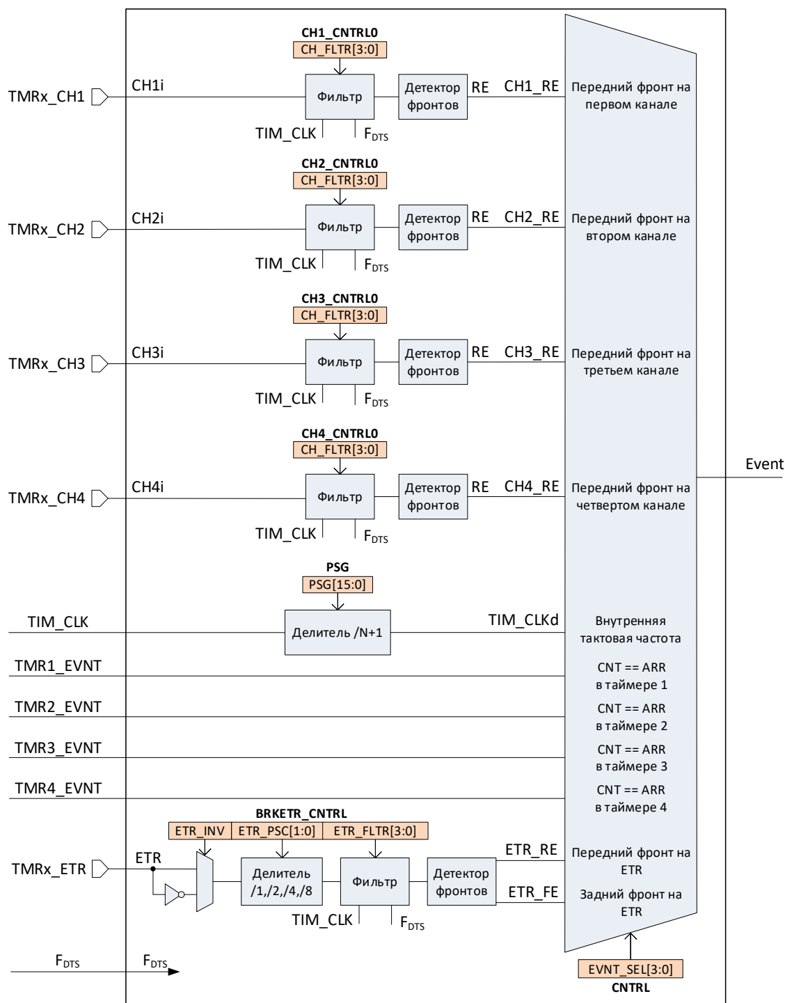
Рисунок 58 – Структурная схема формирования события для счета
