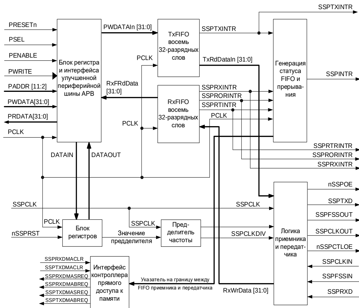
Рисунок 85 – Структурная схема модуля SSP
