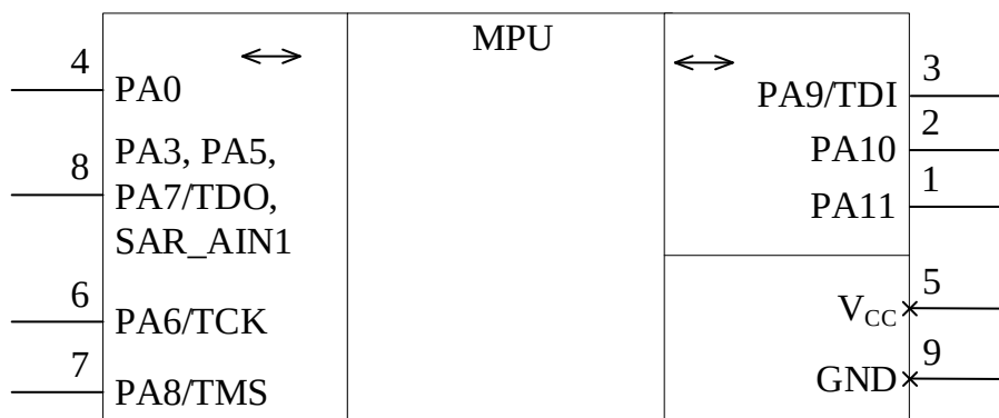
Рисунок 6 – Условное графическое изображение микросхем MDR1219LGI
