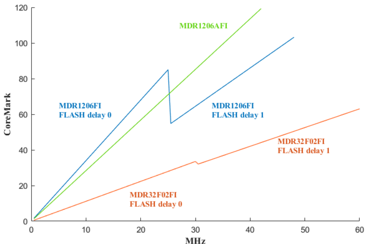
Рисунок 148 – Производительность в Coremark при выполнении из Flash-памяти
