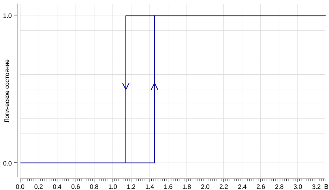
Рисунок 152 – Типовая зависимость логического состояния от напряжения на входе WAKEUP1-WAKEUP3 при U_{CCB} = 3,3 \text{ В} в НУ
