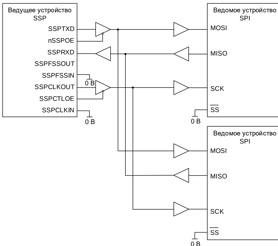
Рисунок 98 – Ведущее устройство SSP подключено к двум ведомым, поддерживающим SPI
