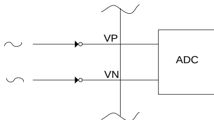
Рисунок 37 – Дифференциальное включение
