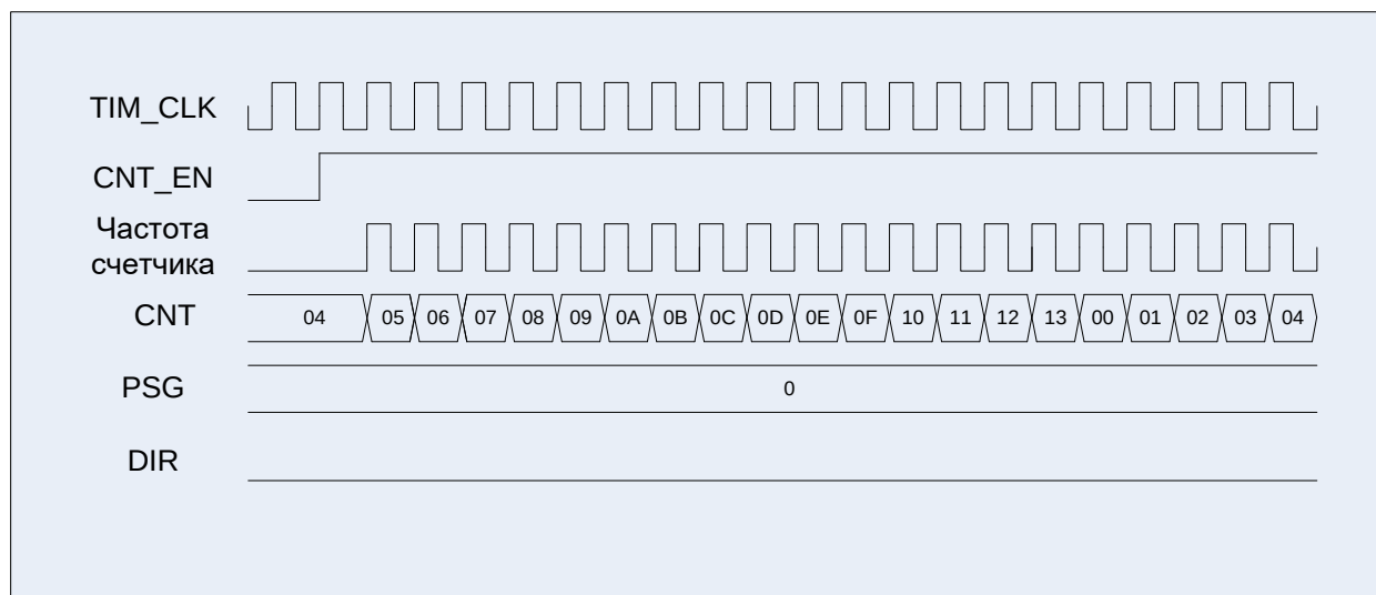
Рисунок 52 – Диаграммы работы таймера, счет прямой от 0 до 0x13, стартовое значение 0x04
