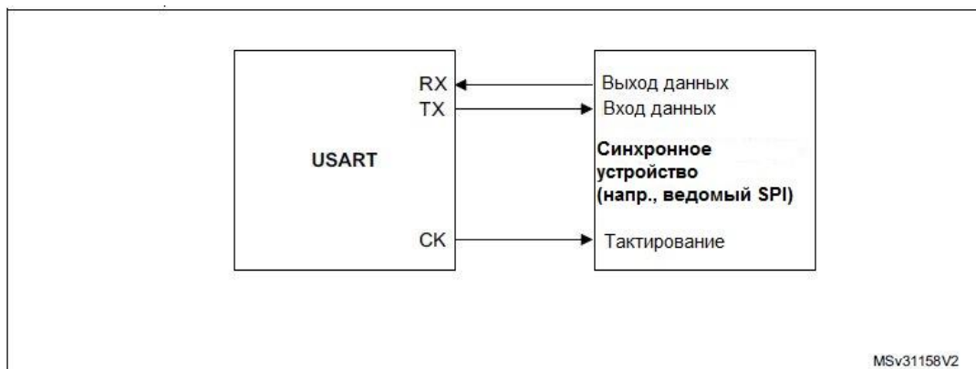
Рисунок 136 – Пример синхронной передачи USART
