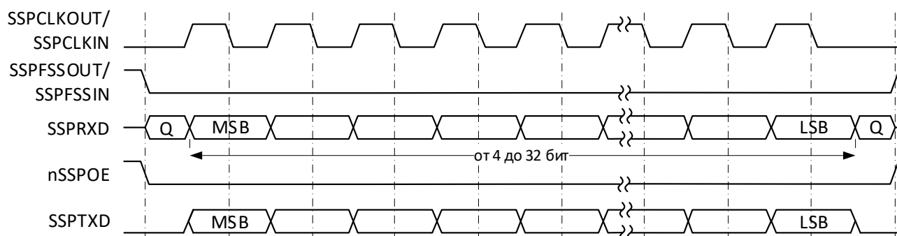
Рисунок 90 – Формат синхронного обмена протокола SPI, SPO=0, SPH=1
