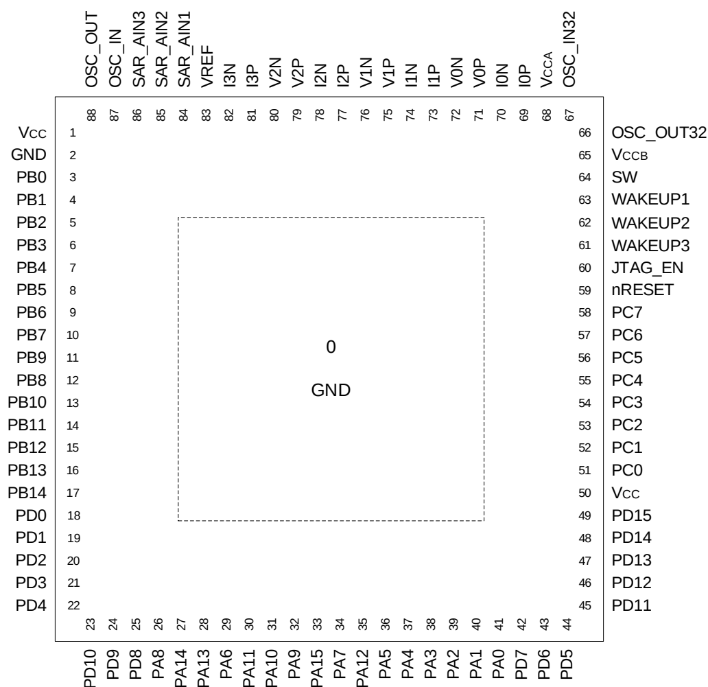
Рисунок 7 – Диаграмма расположения выводов микросхем MDR1206FI, MDR1206AFI
