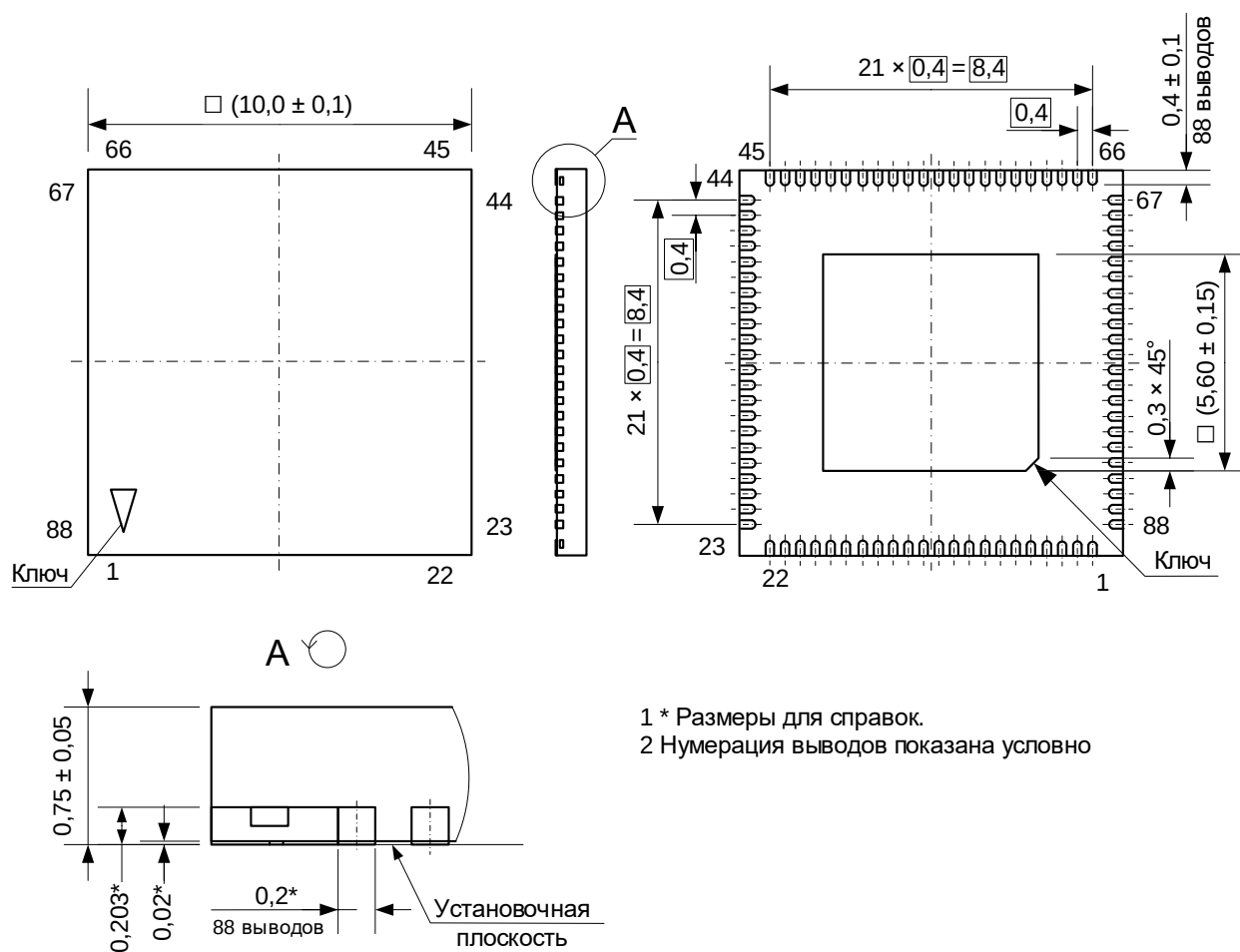
Рисунок 158 – Микросхемы MDR1206FI, MDR1206AFI в корпусе QFN88 10×10×0,75 (0,4)
