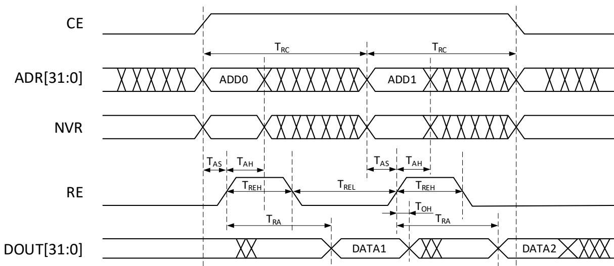
Рисунок 28 – Временная диаграмма чтения памяти
