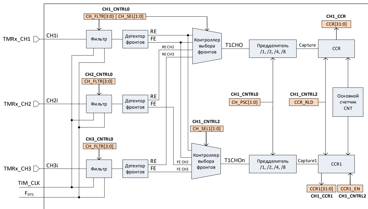
Рисунок 67 – Структурная схема блока захвата на примере канала 1
