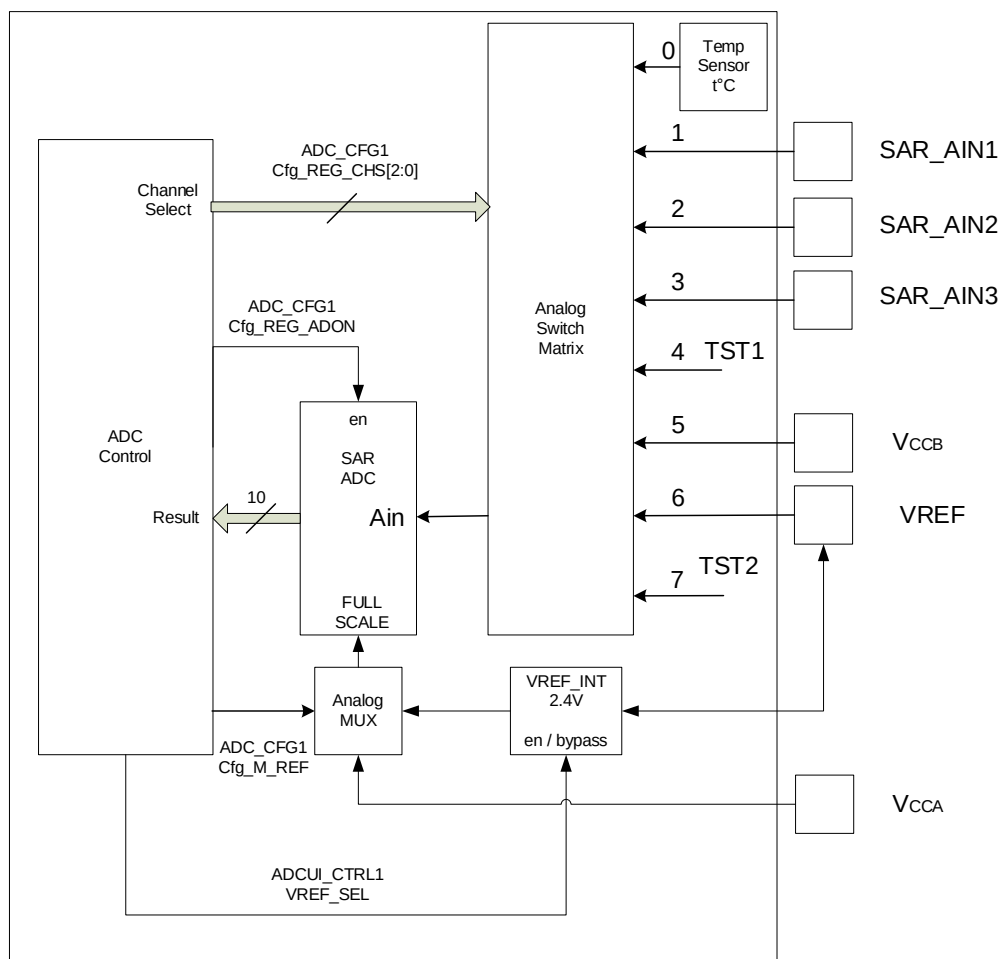
Рисунок 80 – Структурная схема АЦП
