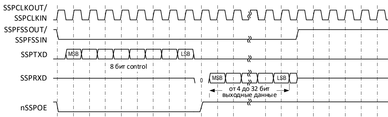
Рисунок 94 – Формат синхронного обмена протокола Microwire (одиночный обмен)
