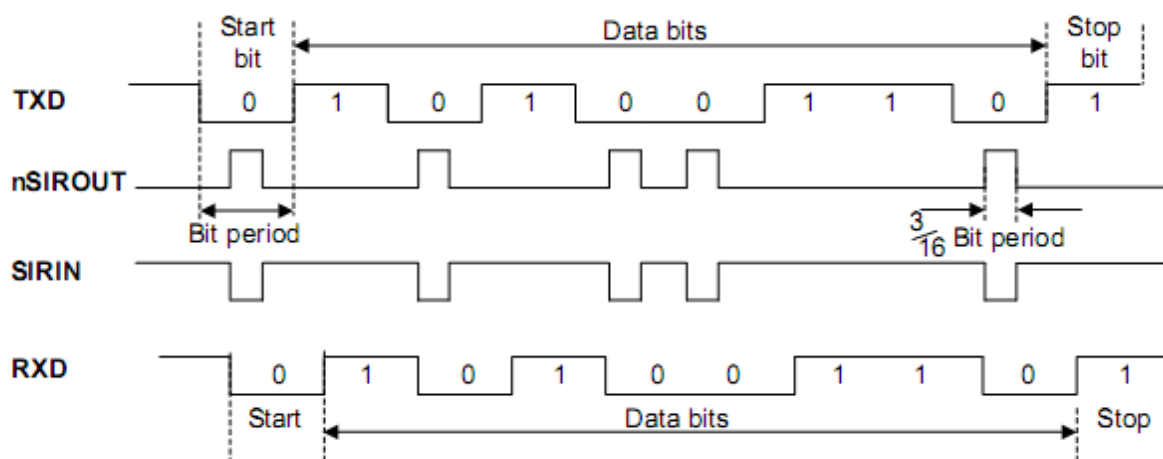
Рисунок 105 – Модуляция данных IrDA
