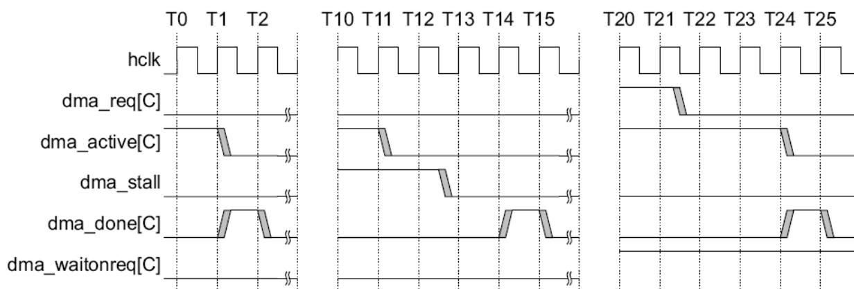
Рисунок 111 – Диаграммы функционирования dma_done
