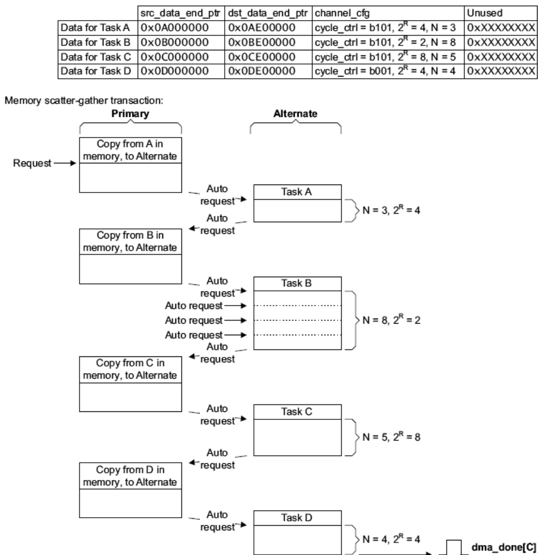
Рисунок 116 – Пример работы DMA в режиме с «Исполнением с изменением конфигурации»
