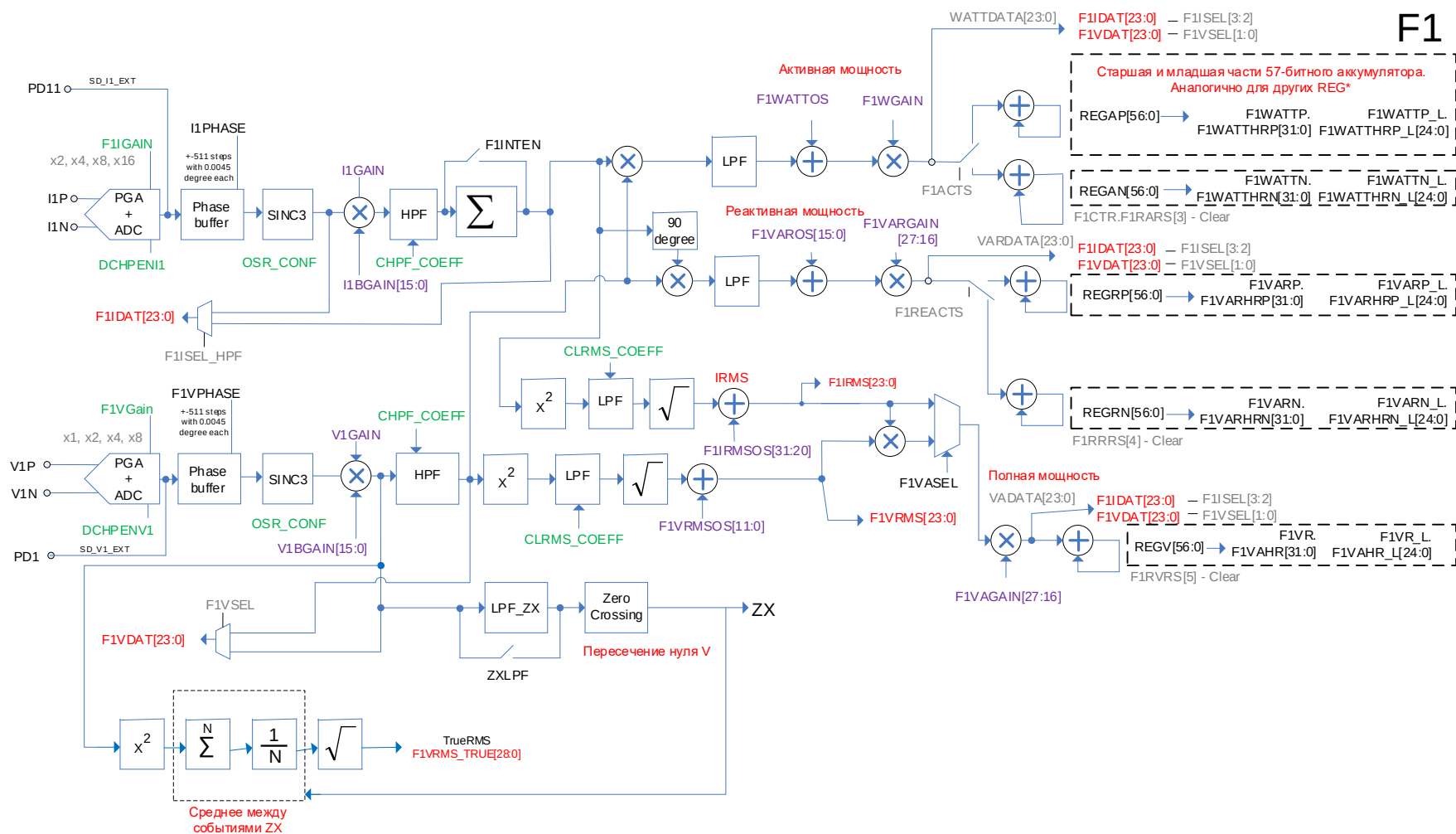
Рисунок 34 – Структурная схема F1
