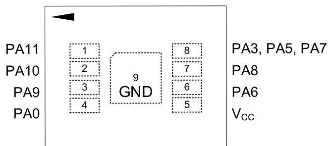
Рисунок 9 – Диаграмма расположения выводов микросхем MDR1219LGI
