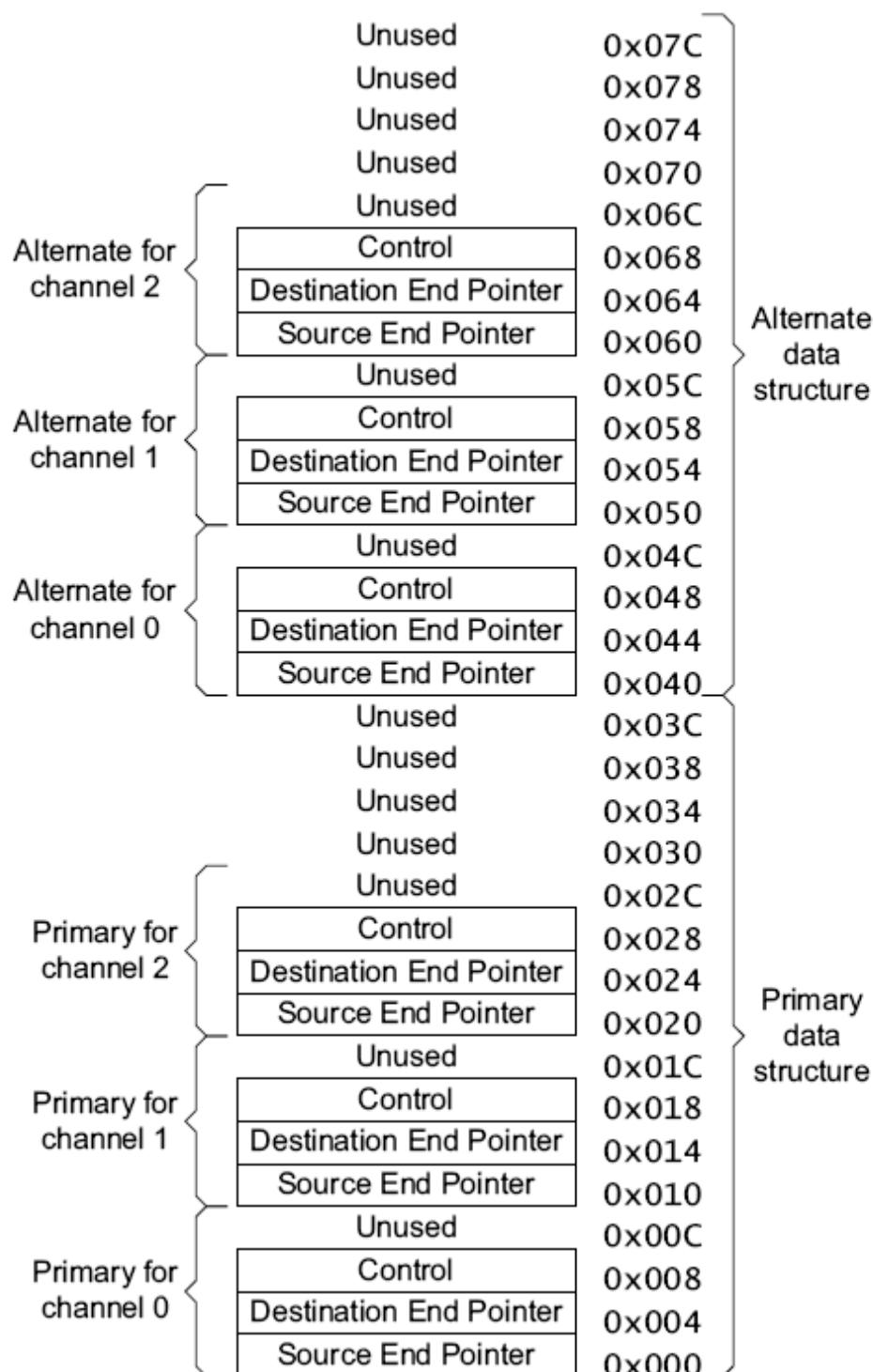
Рисунок 119 – Карта памяти для трех каналов DMA, включая альтернативную структуру управляющих данных (где Destination end pointer – указатель конца данных приемника; Source end pointer – указатель конца данных источника; Control – управление)
