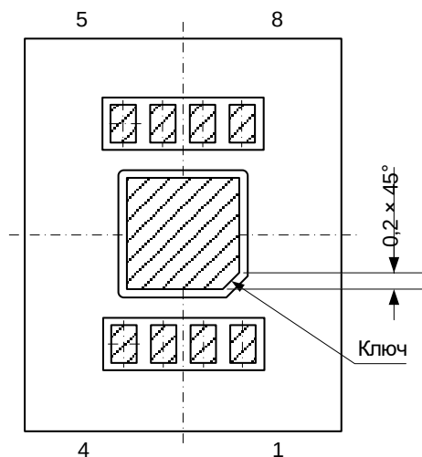
Рисунок 159 – Микросхемы MDR1215LGI в корпусе LGA8 4×5×1,6 (0,5), микросхемы MDR1219LGI в корпусе LGA8 4×5×1,6 (0,5)A
