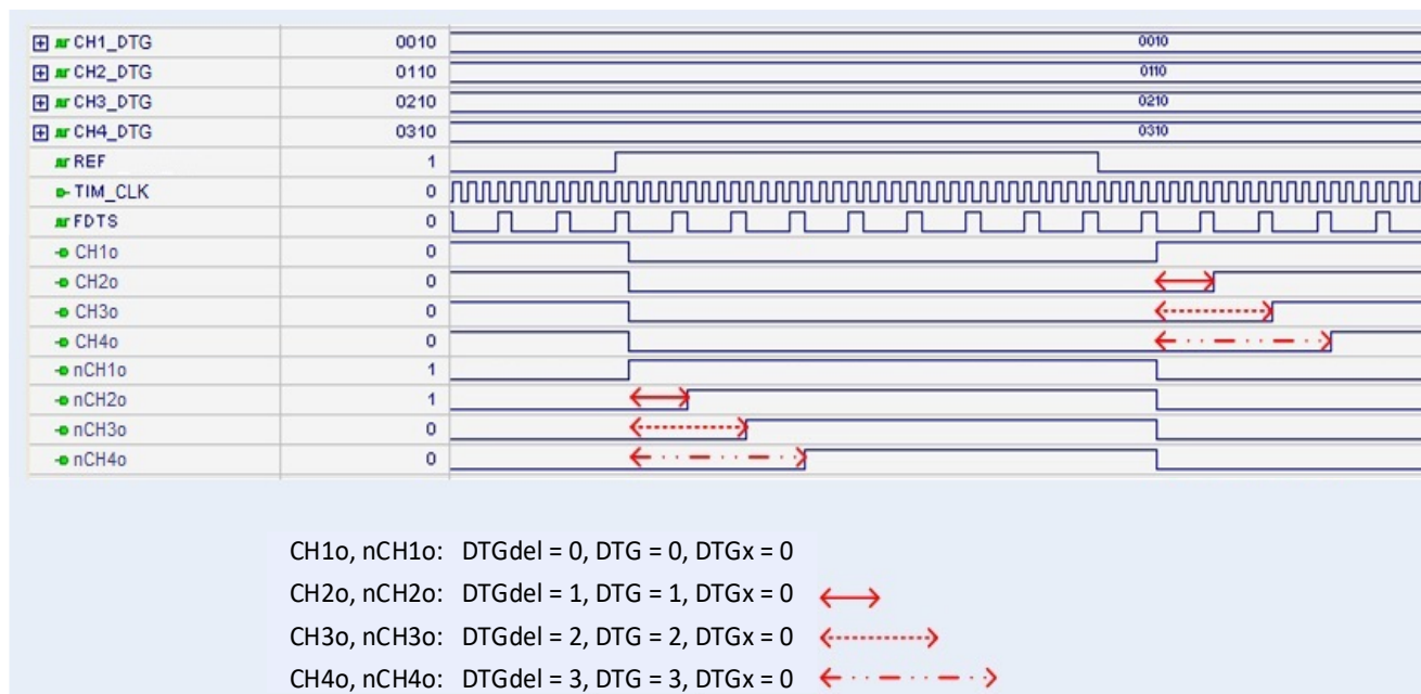
Рисунок 74 – Диаграмма работы блока DTG
