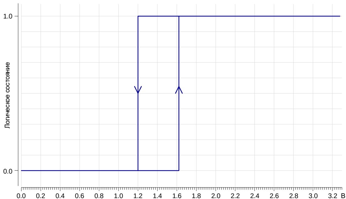
Рисунок 151 – Типовая зависимость логического состояния от напряжения на цифровом входе порта ввода-вывода при U_{CC} = 3,3 В в НУ
