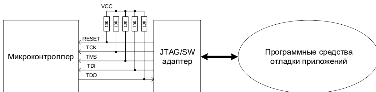
Рисунок 122 – Схема работы в режиме отладки
