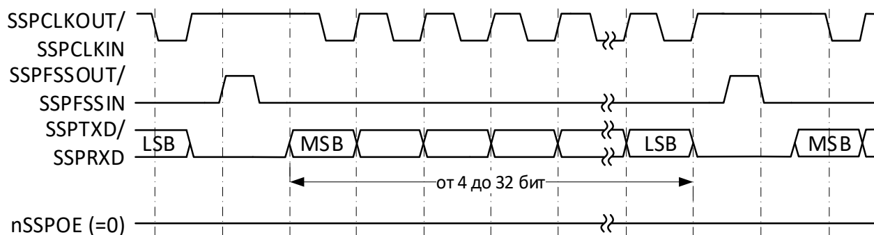
Рисунок 92 – Формат синхронного обмена протокола SPI, SPO=1, SPH=0 (непрерывный обмен)
