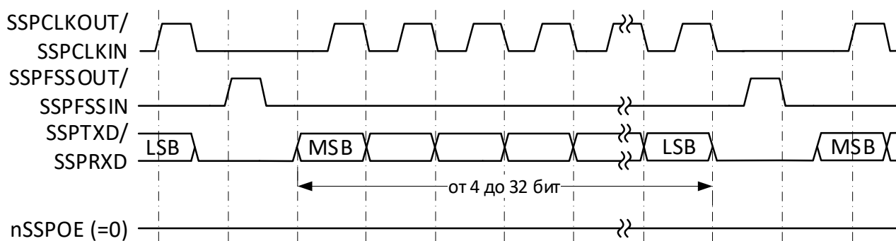
Рисунок 89 – Формат синхронного обмена протокола SPI, SPO=0, SPH=0 (непрерывный обмен)
