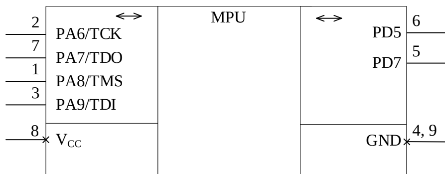
Рисунок 5 – Условное графическое изображение микросхем MDR1215LGI
