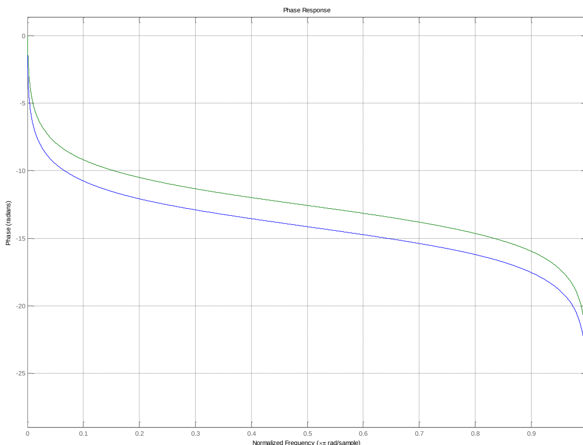
Рисунок 42 – Фильтр для сдвига сигнала на 90^\circ
