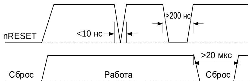
Рисунок 16 – Диаграмма фильтрации помех при формировании сигнала сброса
