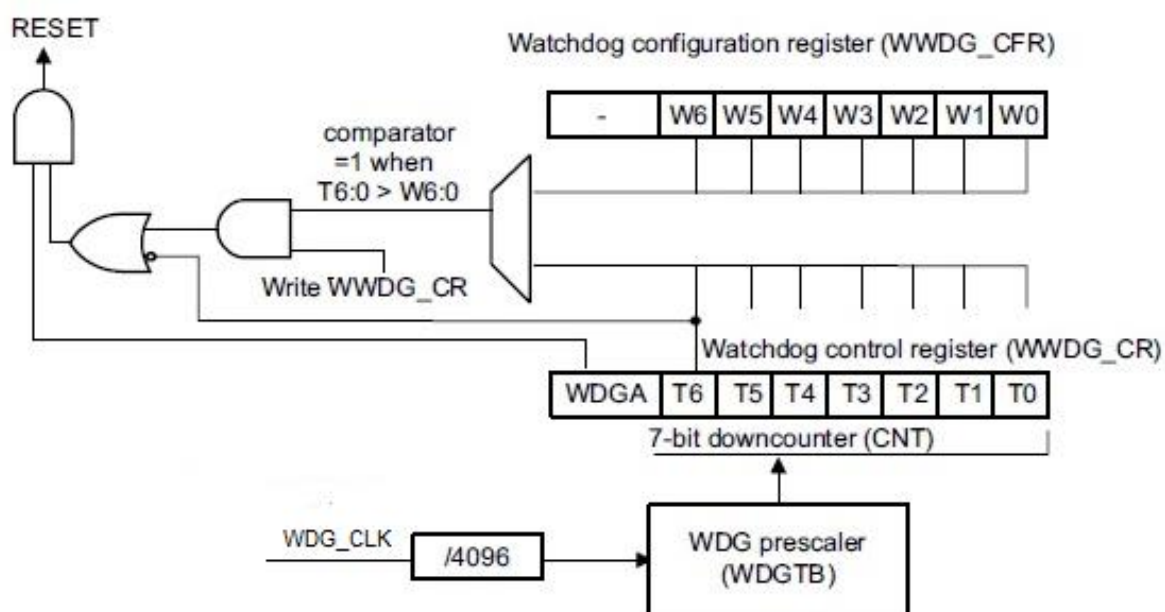
Рисунок 124 – Блок-схема оконного сторожевого таймера
