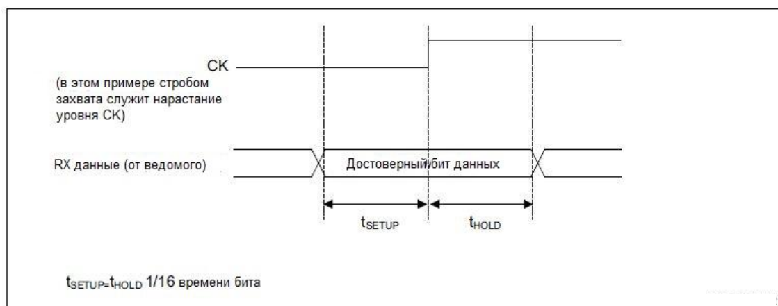
Рисунок 139 – Время установки/удержания RX
