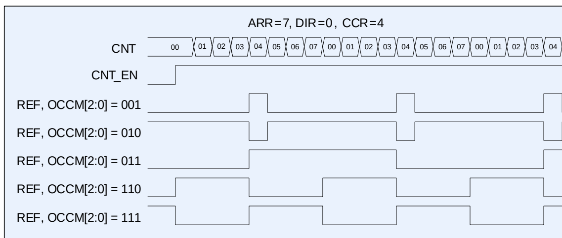
Рисунок 70 – Диаграмма работы в режиме ШИМ, CCR1_EN=0
