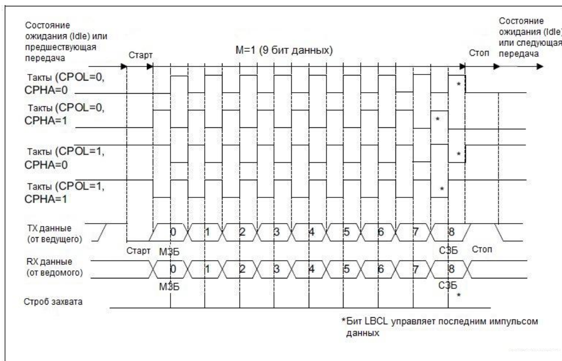
Рисунок 138 – Диаграмма тактирования данных USART (M=1)
