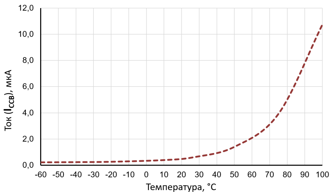
Рисунок 155 – Зависимость статического тока потребления I_{CCB} батарейного домена микросхем MDR1206FI (CHIP_ID = 217) от температуры при U_{CCB} = 3,3 В и отсутствии основного питания
