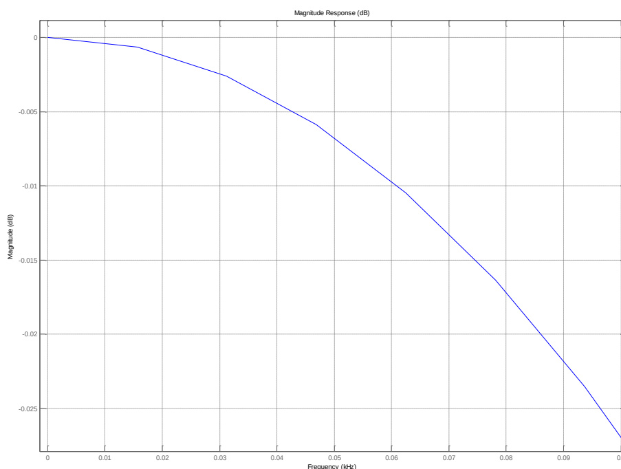
Рисунок 41 – Характеристика децимирующего фильтра в полосе 100 Гц при настройках по умолчанию
