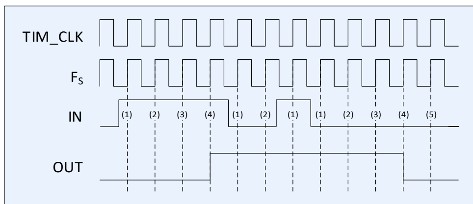
Рисунок 75 – Диаграмма работы фильтра, F_S = \text{TIM\_CLK} , N = 4
