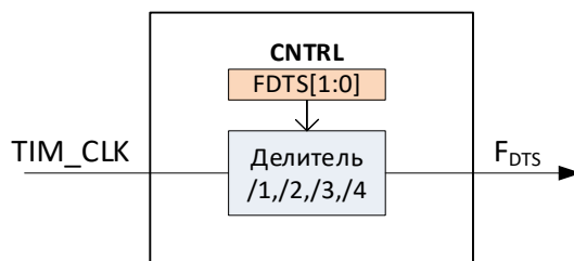
Рисунок 56 – Схема формирования тактовой частоты F DTS
