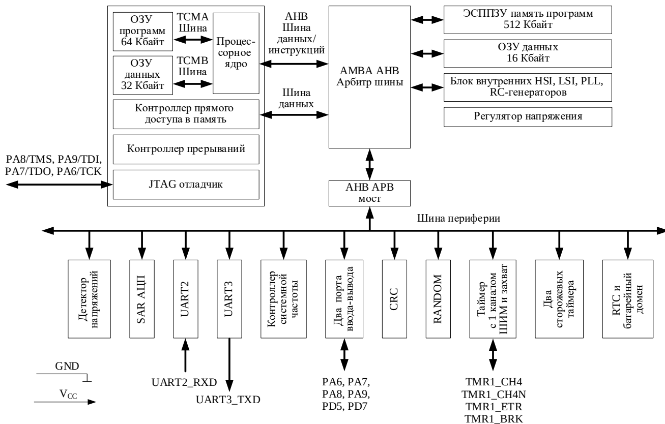
Рисунок 2 – Структурная блок-схема микросхем MDR1215LGI
