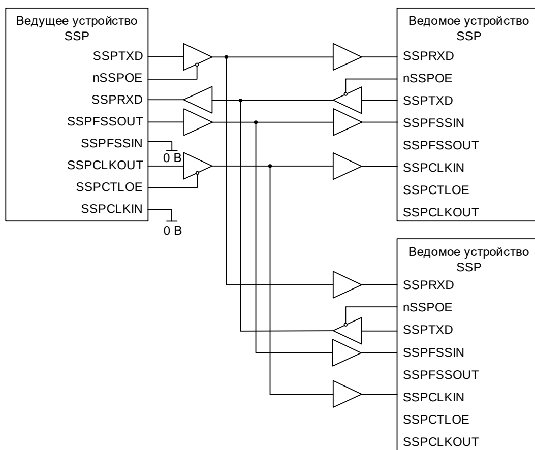
Рисунок 97 – Ведущее устройство SSP подключено к двум ведомым
