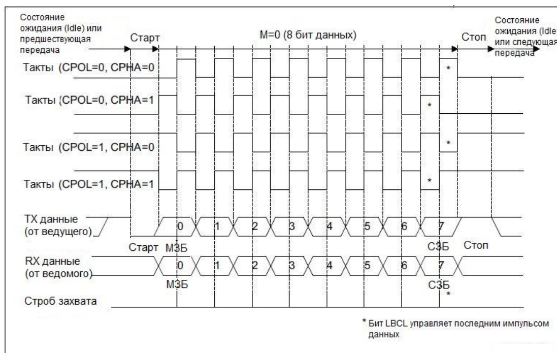
Рисунок 137 – Диаграмма тактирования данных USART (M=0)
