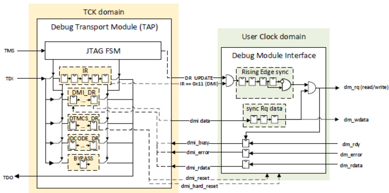
Рисунок 121 – Интерфейс DM
