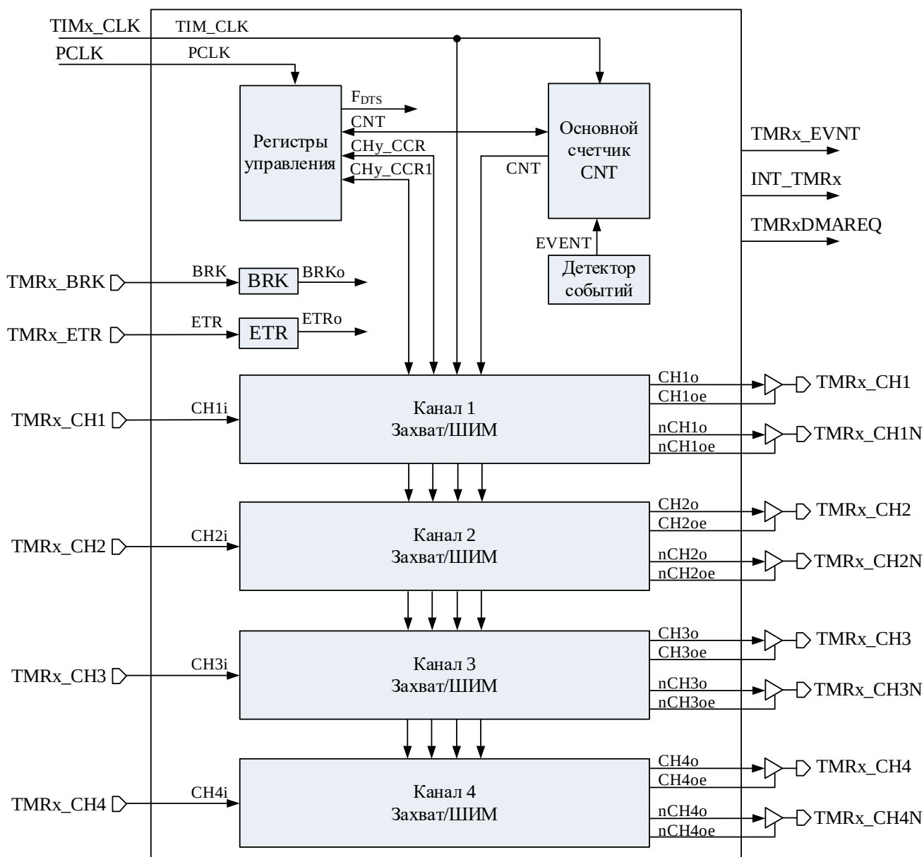
Рисунок 51 – Структурная схема блока «Таймер»
