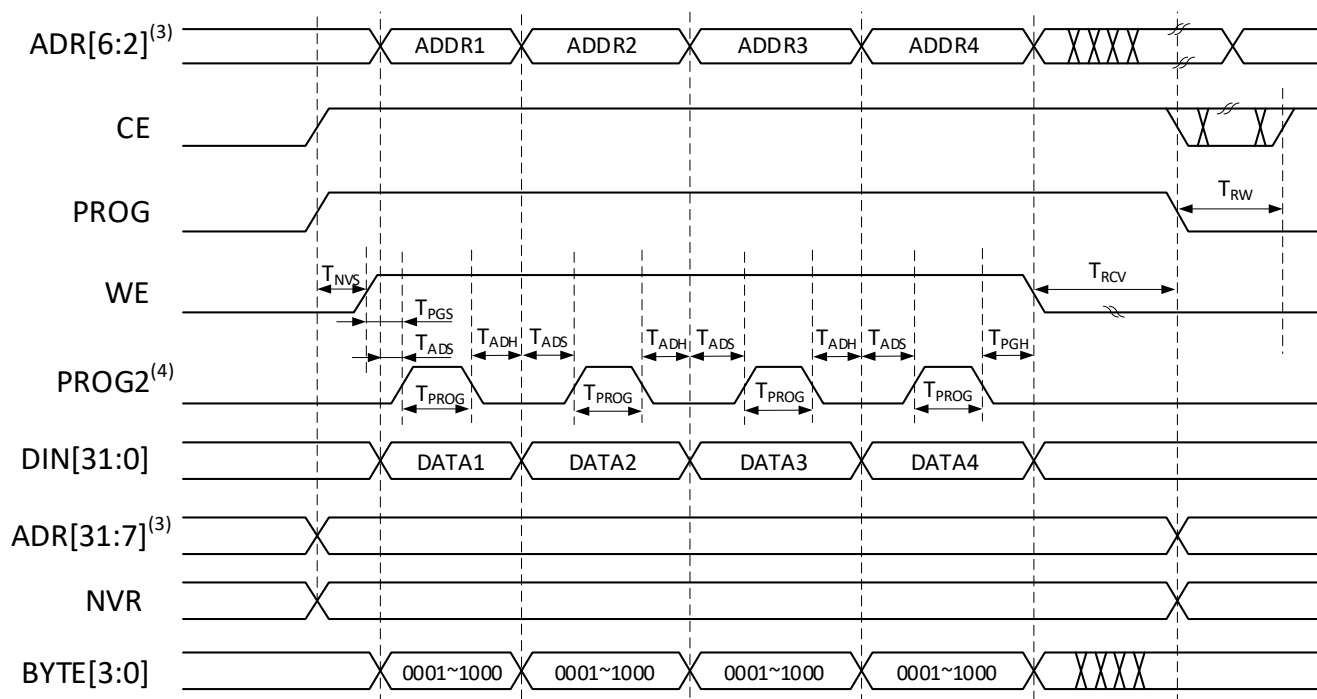
Рисунок 27 – Временная диаграмма записи памяти
