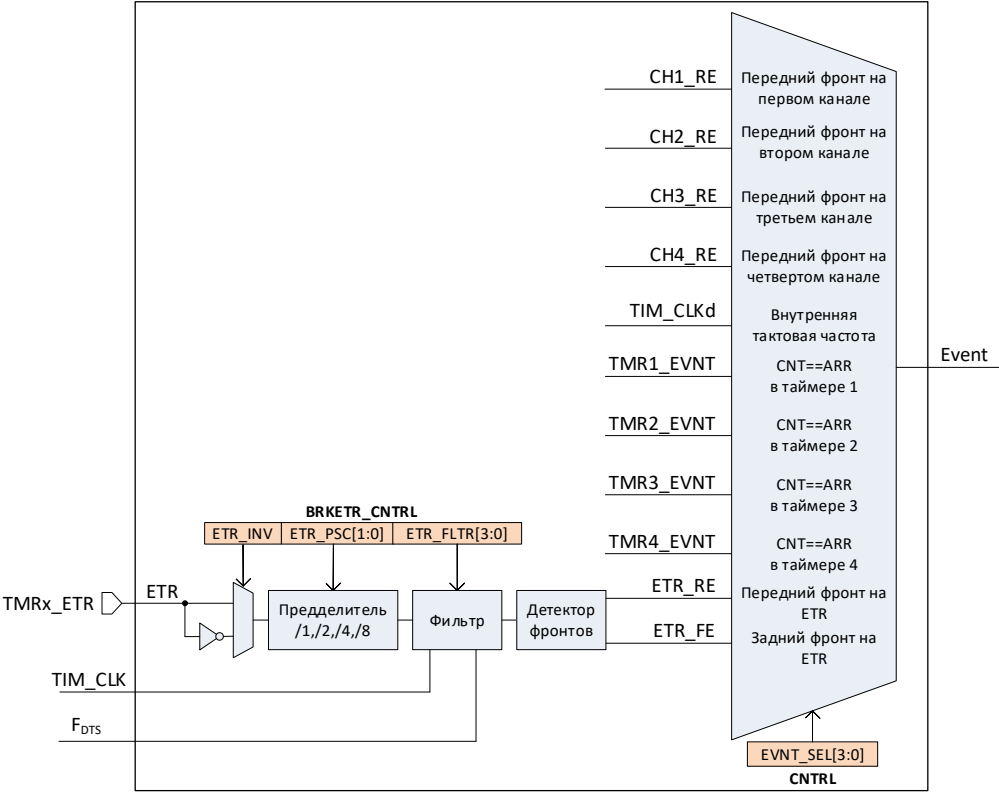
Рисунок 65 – Схема тактирования сигналом со входа ETR
