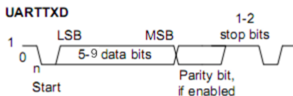
Рисунок 104 – Кадр передачи данных
