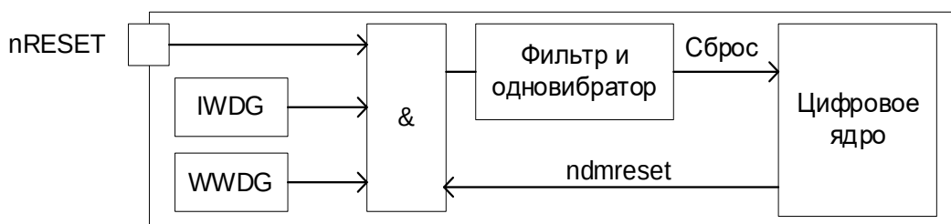
Рисунок 15 – Блок-схема формирования сброса
