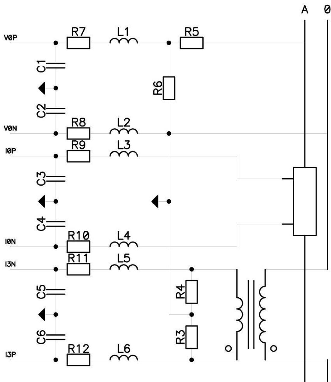
Рисунок 45 – Типовая схема включения для учета электроэнергии по одной фазе с использованием шунта
