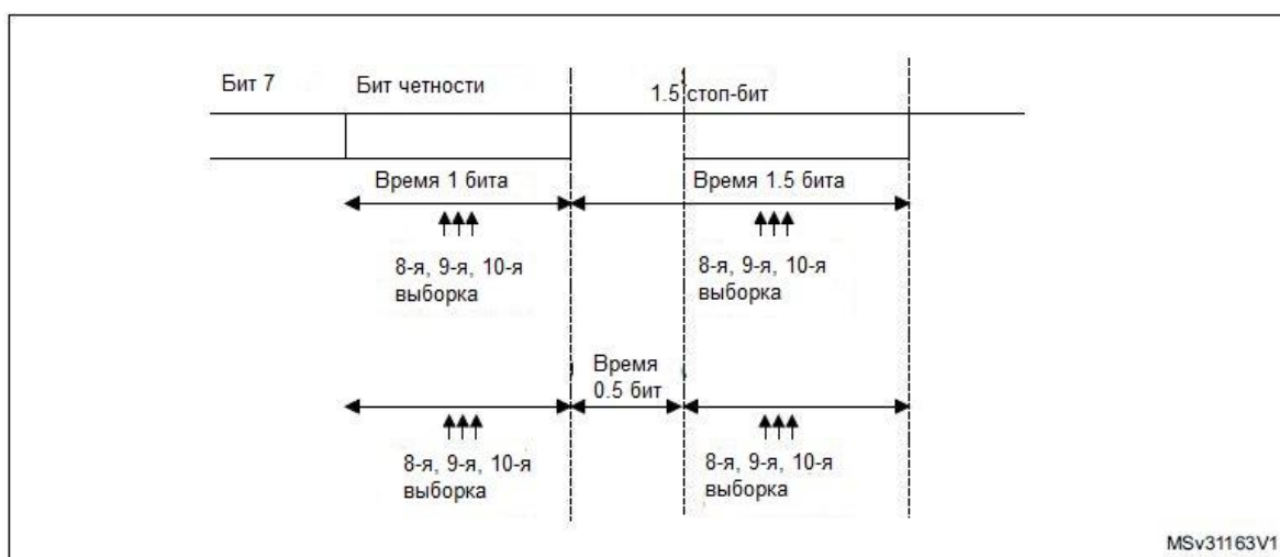
Рисунок 141 – Обнаружение ошибки четности с использованием 1,5 стоп-бит
